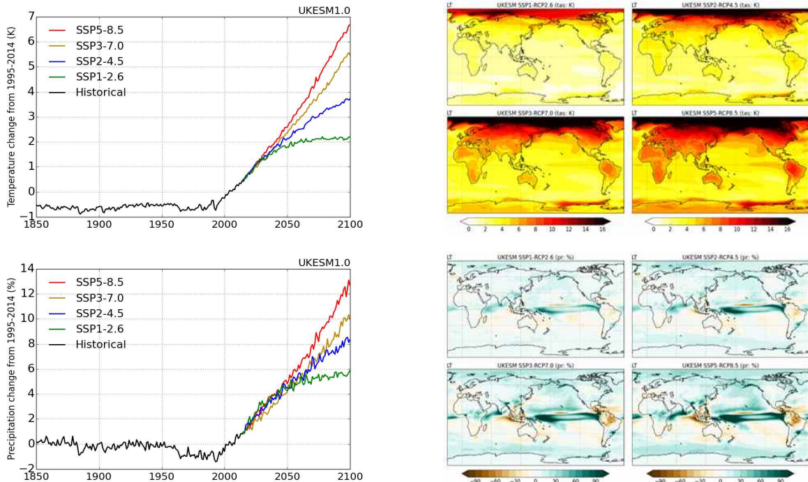
그림 2. 신규 기후변화 시나리오기반의 평균 기온과 강수량의 미래전망 시계열(좌)과 4종 시나리오에 따른 21세기 후반기(2081~2100)의 전지구 평균기온과 강수량의 수평분포(우)
