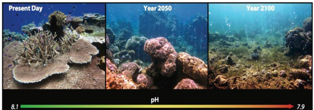
<파푸아 뉴기니의 이산화탄소 분압(pCO 2 )와 수소이온농도(pH) 분포에 따른 해양산성화>
