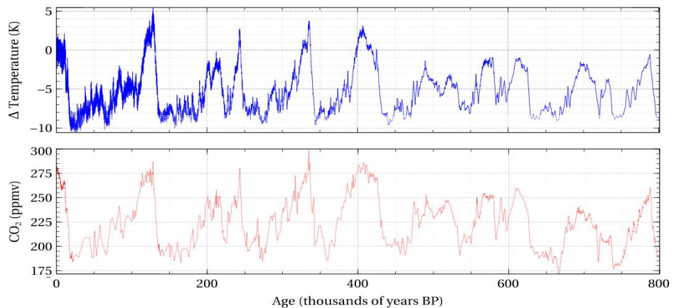
<남극 빙하코어의 80만년간 평균기온과 이산화탄소 농도 변화> [출처: By Fabrice.Lambert, https://commons.wikimedia.org ]
