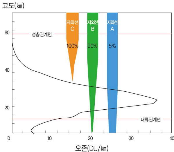
<성층권에서 자외선 흡수량 >
