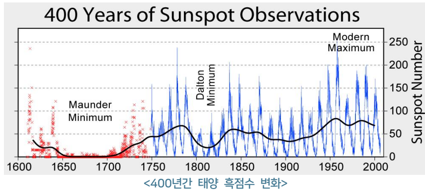
<400년간 태양 흑점수 변화> [출처 : Robert A. Rohde, Global Warming Art Project.]
