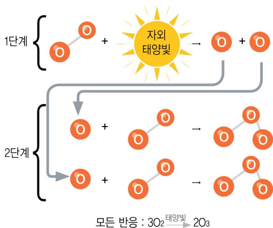
<성층권 오존의 생성>
