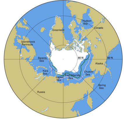
<북극 해빙의 면적 변화(좌 : 1989년 9월, 우 : 2019년 9월)> 분홍색선: 30년 평균('90~'19), 녹색선: 10년평균('10~'19)
