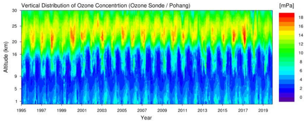
<포항지역의 오존농도 연직분포(1995~2019년)>
