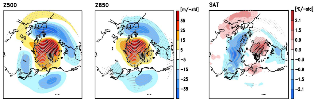
<음의 북극진동 시 북극해와 우리나라 주변 500hPa, 850hPa 지위고도, 지상기온(SAT) 패턴>
