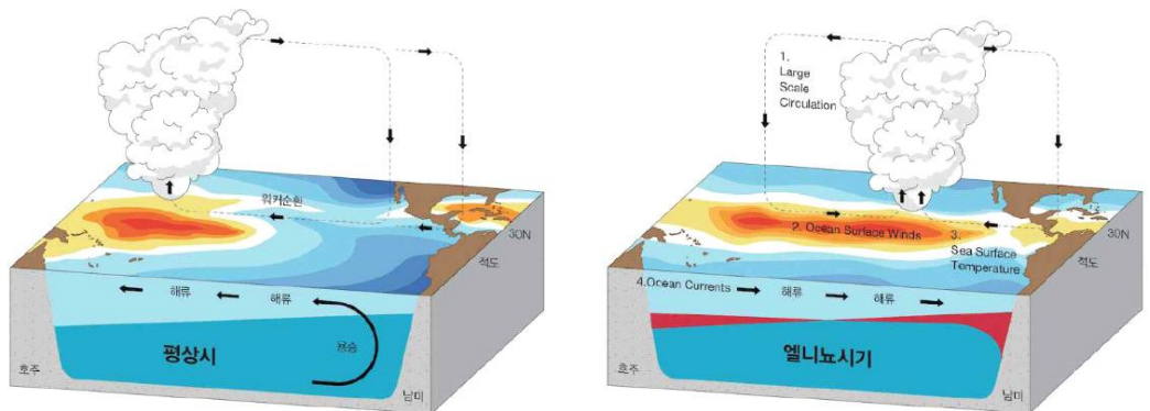
<평상시와 엘니뇨 시기 대기·해양 모식도>
