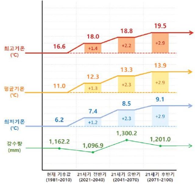
RCP4.5
