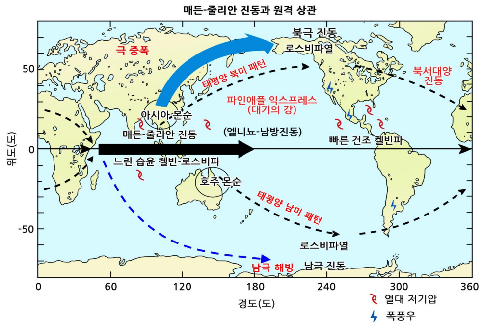
<MJO와 원격상관의 도식화(서경환 등, 기후역학교과서, 2017)>
