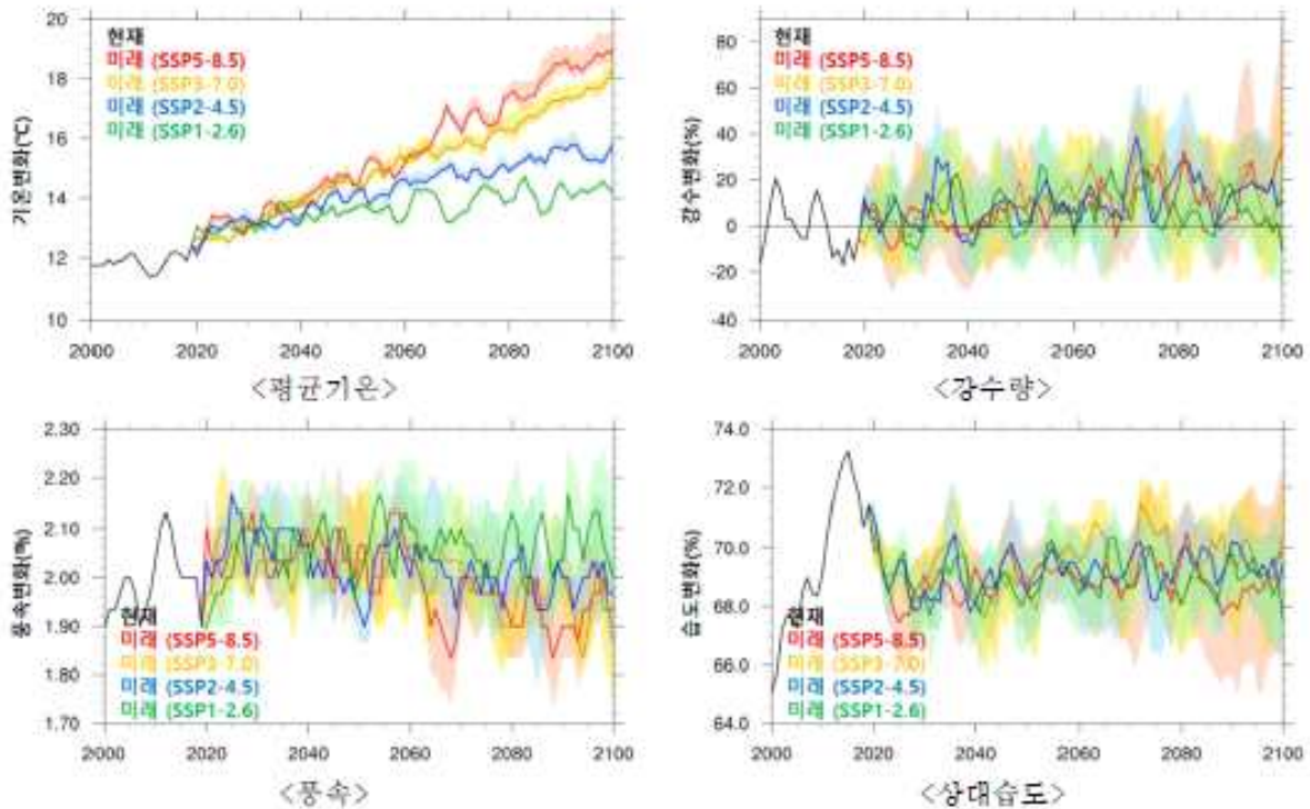
<SSP 기반, 현재(2000~2019년) 대비 2000~2100년의 우리나라 기온, 강수량, 풍속, 상대습도 변화>
