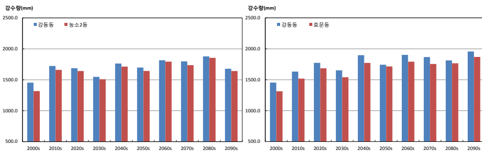
그림 3-5. 연강수량(mm) 증가율이 가장 큰 지역 (농소2동, 효문동)과 작은 지역(강동동)의 시계열 (RCP4.5(좌), RCP8.5(우))
