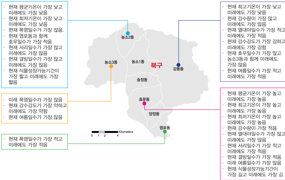
그림 5-1. 울산광역시 북구의 동별 기후변화 전망 요약
