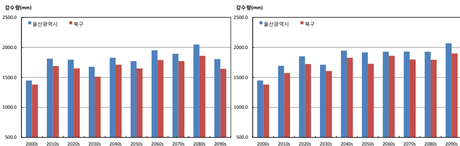
그림 3-4. 울산광역시와 북구의 연강수량(mm) 시계열 (RCP4.5(좌), RCP8.5(우))
