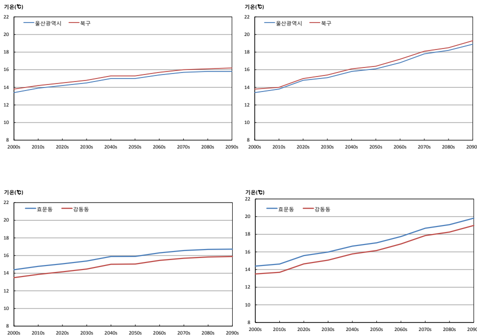
그림 3-1. 울산광역시와 북구의 평균기온(℃) 시계열(RCP4.5(좌), RCP8.5(우))
