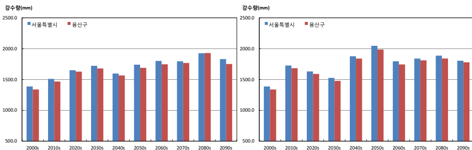
그림 3-4. 서울특별시와 용산구의 연강수량(mm) 시계열 (RCP4.5(좌), RCP8.5(우))
