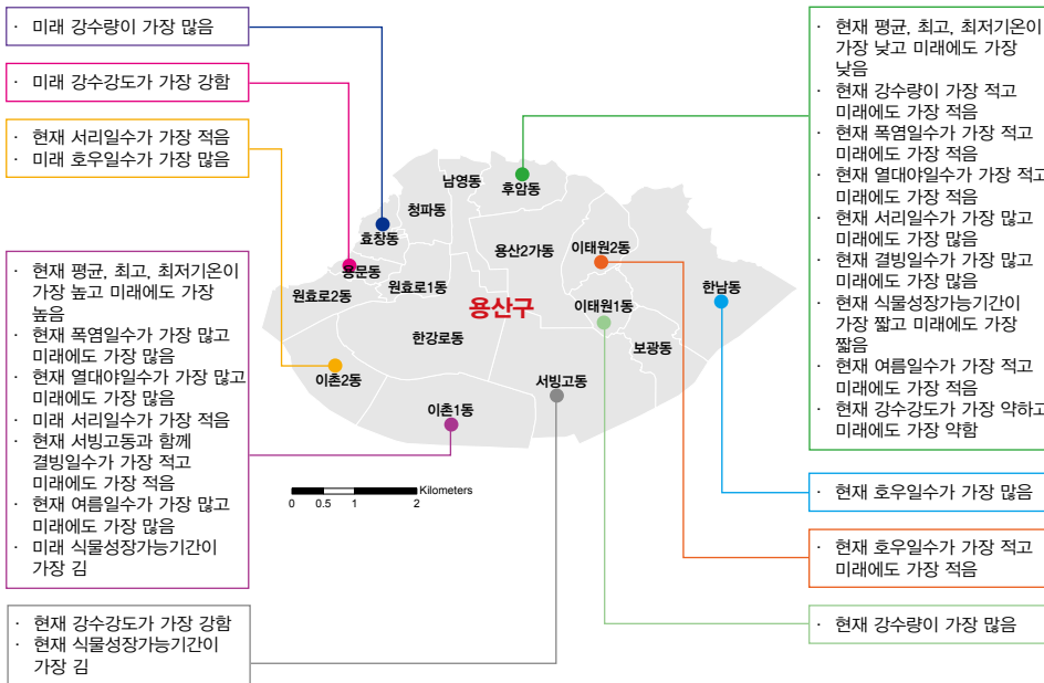
그림 5-1. 서울특별시 용산구의 동별 기후변화 전망 요약(RCP8.5 2071~2100년)
