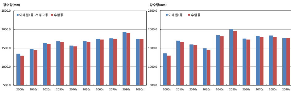
그림 3-5. 연강수량(mm) 증가율이 가장 큰 지역(주암동)과 작은 지역(이태원1동, 서빙고동)의 시계열(RCP4.5(좌), RCP8.5(우))
