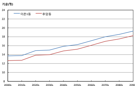
그림 3-2. 평균기온(℃) 증가율이 가장 큰 지역 (이태원1동, 후암동)과 작은 지역(이촌1동)의 시계열(RCP4.5(좌), RCP8.5(우))
