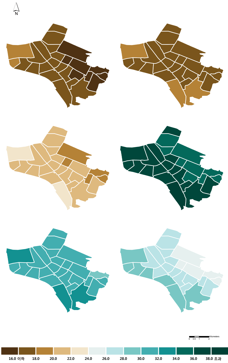
그림 3-7. 송파구의 동별 강수량 증가율(%) (2001~2010년 대비) 분포도 (RCP4.5(좌)/8.5(우), 2011~2040년(상), 2041~2070년(중), 2071~2100년(하))
