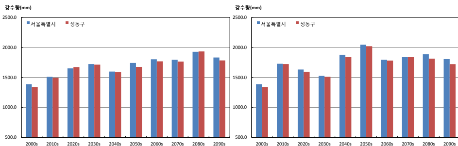
그림 3-4. 서울특별시와 성동구의 연강수량(mm) 시계열 (RCP4.5(좌), RCP8.5(우))
