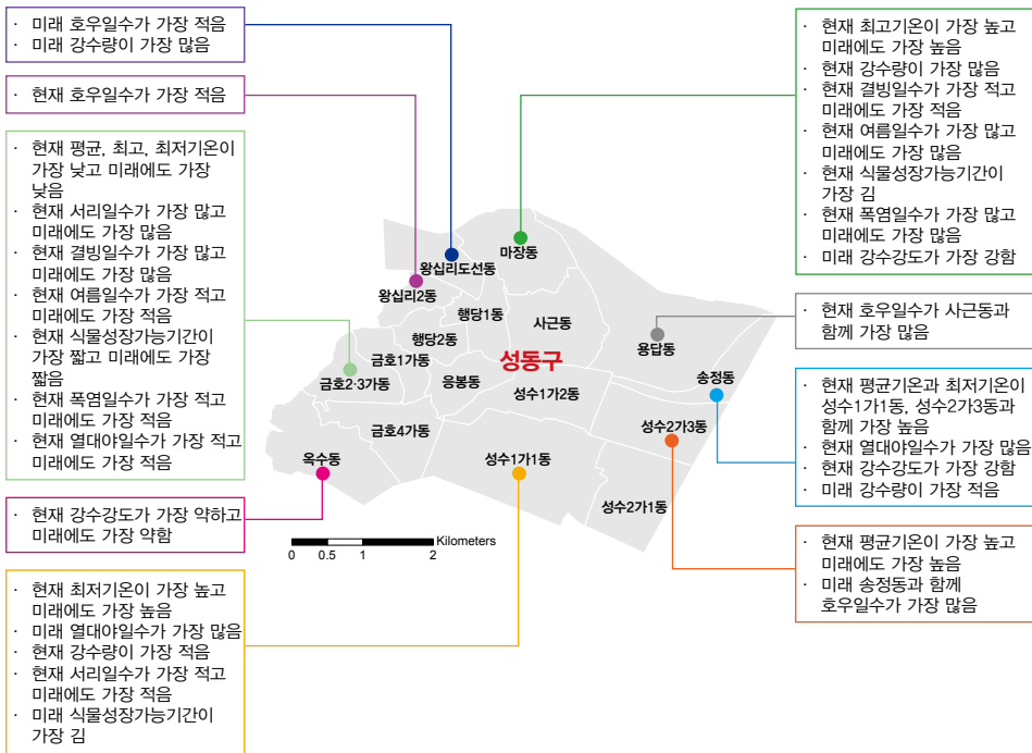
그림 5-1. 서울특별시 성동구의 동별 기후변화 전망 요약(RCP8.5 2071~2100년)
