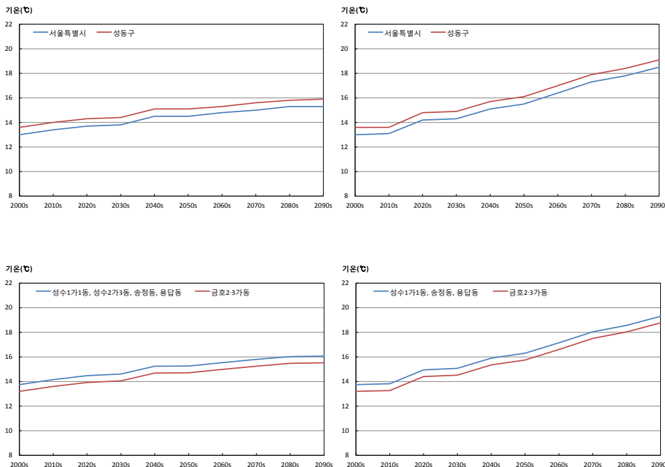
그림 3-1. 서울특별시와 성동구의 평균기온(℃) 시계열(RCP4.5(좌), RCP8.5(우))
