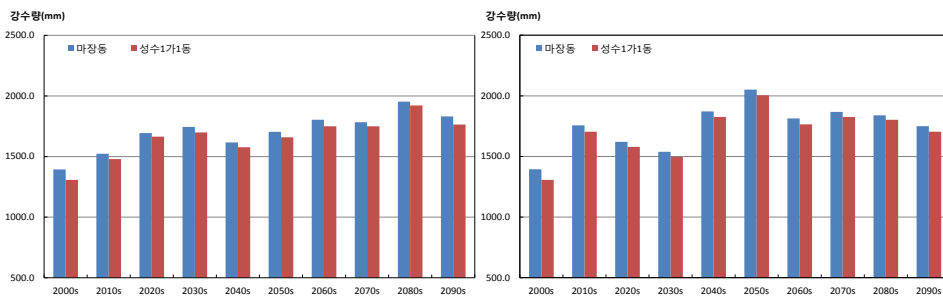
그림 3-5. 연강수량(mm) 증가율이 가장 큰 지역 (성수1가1동)과 작은 지역(마장동)의 시계열(RCP4.5(좌), RCP8.5(우))
