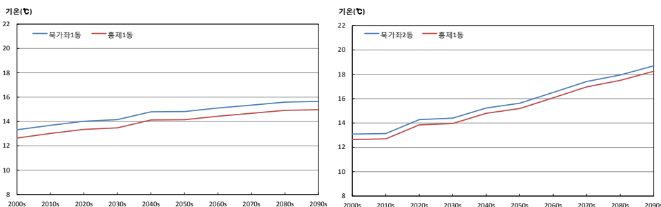
그림 3-2. 평균기온(℃) 증가율이 가장 큰 지역(홍제1동)과 작은 지역(북가좌1동, 북가좌2동)의 시계열(RCP4.5(좌), RCP8.5(우))
