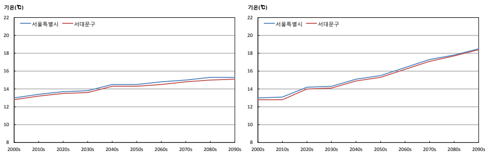
그림 3-1. 서울특별시와 서대문구의 평균기온(℃) 시계열(RCP4.5(좌), RCP8.5(우))
