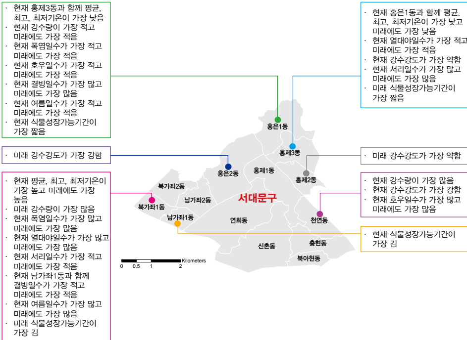
그림 5-1. 서울특별시 서대문구의 동별 기후변화 전망 요약(RCP8.5 2071~2100년)
