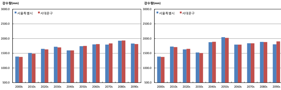
그림 3-4. 서울특별시와 서대문구의 연강수량(mm) 시계열 (RCP4.5(좌), RCP8.5(우))
