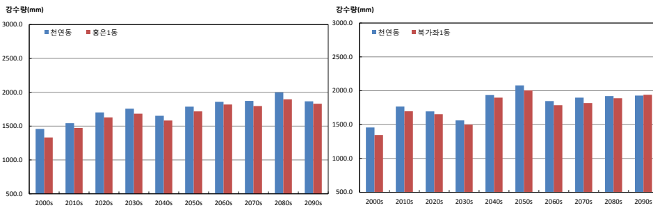
그림 3-5. 연강수량(mm) 증가율이 가장 큰 지역 (홍은1동, 북가좌1동)과 작은 지역(천연동)의 시계열(RCP4.5(좌), RCP8.5(우))
