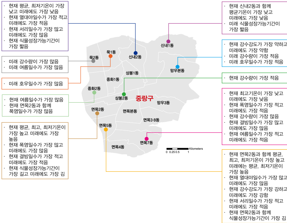
그림 5-1. 서울특별시 중랑구의 동별 기후변화 전망 요약(RCP8.5 2071~2100년)
