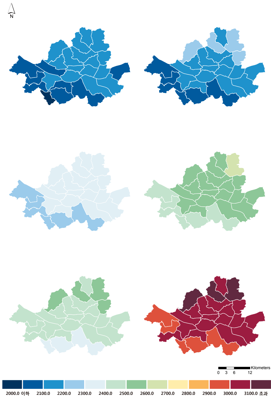
그림 4-2. 서울특별시 구별 유효적산온도(10°C)(°C) 분포도 (RCP4.5(좌)/8.5(우), 2011~2040년(상), 2041~2070년(중), 2071~2100년(하))
