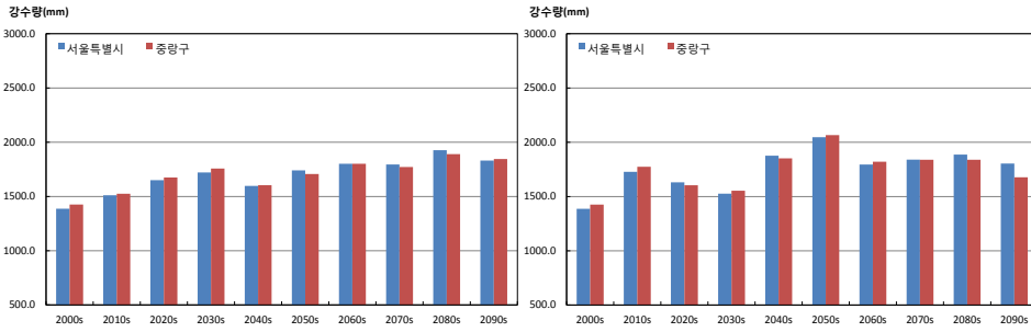
그림 3-4. 서울특별시와 중랑구의 연강수량(mm) 시계열 (RCP4.5(좌), RCP8.5(우))
