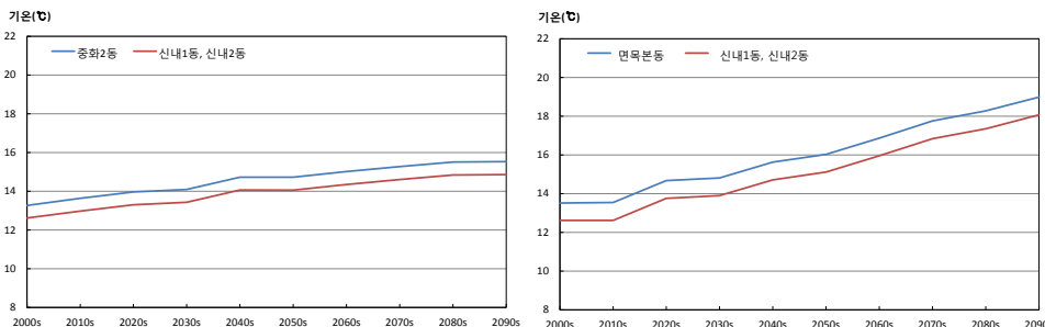
그림 3-2. 평균기온(℃) 증가율이 가장 큰 지역(신내1동, 신내2동)과 작은 지역(중화2동, 면목본동)의 시계열(RCP4.5(좌), RCP8.5(우))
