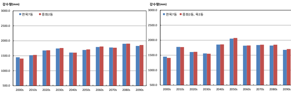
그림 3-5. 연강수량(mm) 증가율이 가장 큰 지역 (중화2동, 목2동)과 작은 지역(면목7동)의 시계열(RCP4.5(좌), RCP8.5(우))
