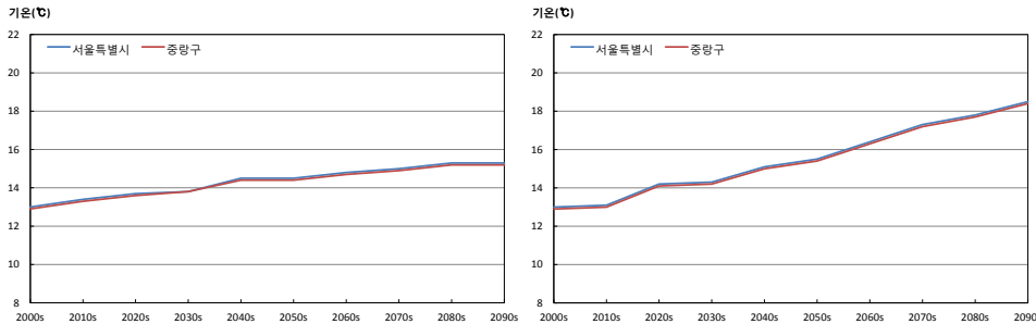
그림 3-1. 서울특별시와 중랑구의 평균기온(℃) 시계열(RCP4.5(좌), RCP8.5(우))
