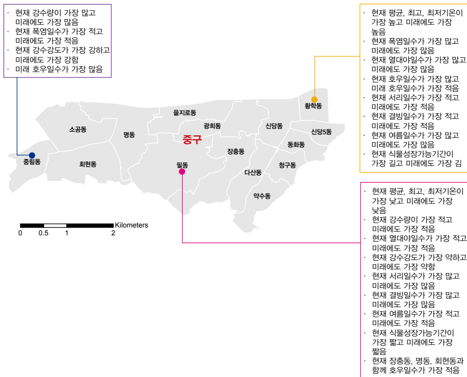
그림 5-1. 서울특별시 중구의 동별 기후변화 전망 요약(RCP8.5 2071~2100년)
