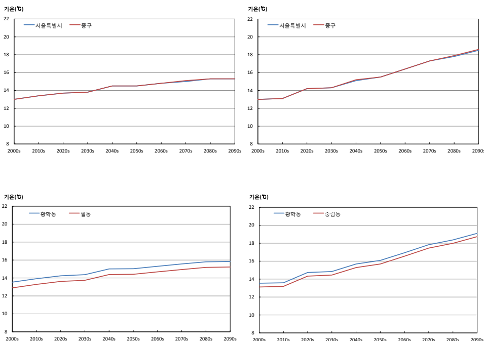
그림 3-1. 서울특별시와 중구의 평균기온(℃) 시계열(RCP4.5(좌), RCP8.5(우))
