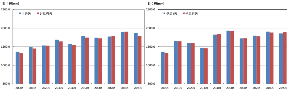
그림 3-5. 연강수량(mm) 증가율이 가장 큰 지역(신도림동)과 작은 지역(수궁동, 구로4동)의 시계열(RCP4.5(좌), RCP8.5(우))
