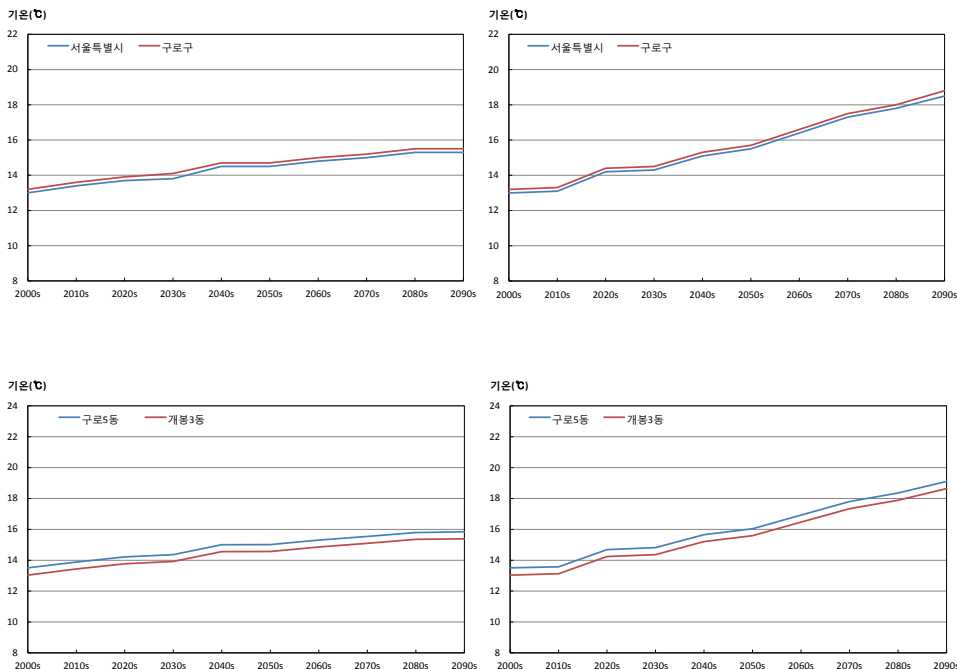
그림 3-1. 서울특별시와 구로구의 평균기온(°C) 시계열(RCP4.5(좌), RCP8.5(우))
