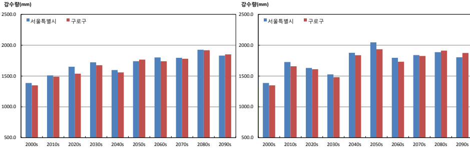
그림 3-4. 서울특별시와 구로구의 연강수량(mm) 시계열 (RCP4.5(좌), RCP8.5(우))
