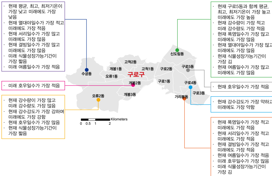
그림 5-1. 서울특별시 구로구의 동별 기후변화 전망 요약(RCP8.5 2071~2100년)
