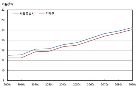
그림 3-1. 서울특별시와 은평구의 평균기온(℃) 시계열(RCP4.5(좌), RCP8.5(우))
