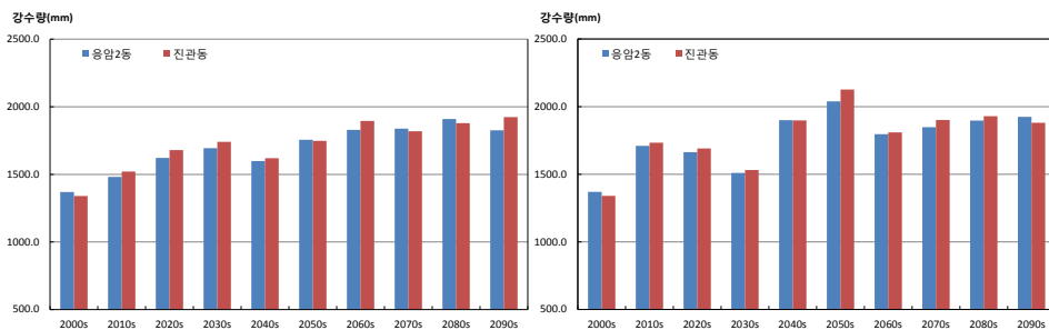
그림 3-5. 연강수량(mm) 증가율이 가장 큰 지역 (진관동)과 작은 지역(응암2동)의 시계열(RCP4.5(좌), RCP8.5(우))
