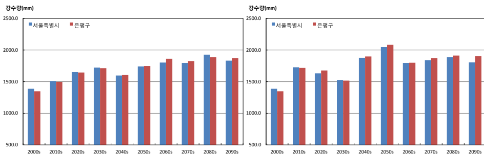
그림 3-4. 서울특별시와 은평구의 연강수량(mm) 시계열 (RCP4.5(좌), RCP8.5(우))
