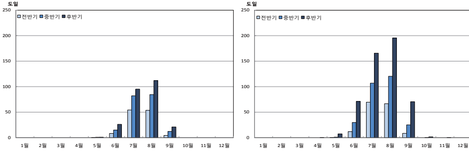
그림 4-1. 세종특별자치시의 월별 냉방도일 전망(RCP4.5(좌), RCP8.5(우))
