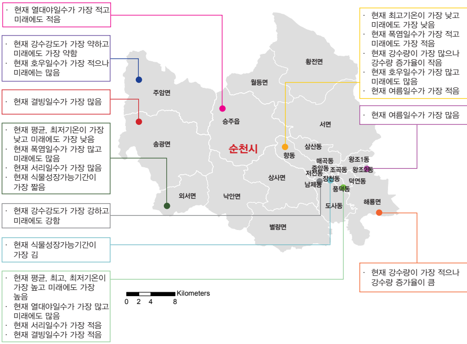
그림 5-1. 전라남도 순천시의 읍면동별 기후변화 전망 요약
