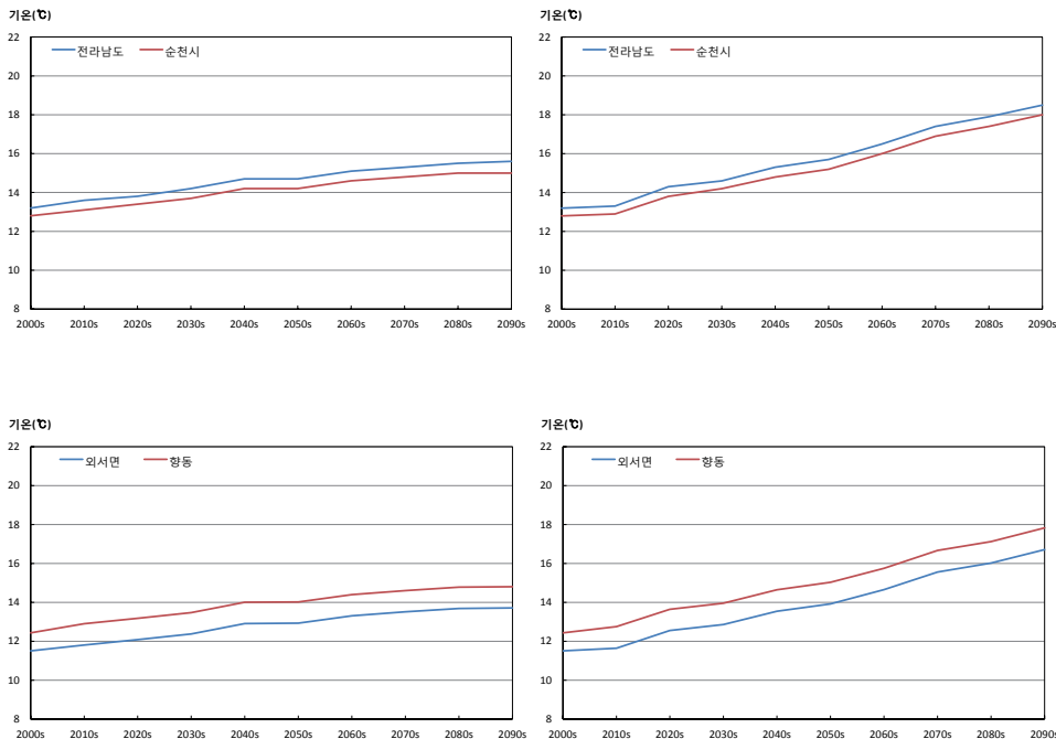
그림 3-1. 전라남도과 순천시의 평균기온(℃) 시계열(RCP4.5(좌), RCP8.5(우))
