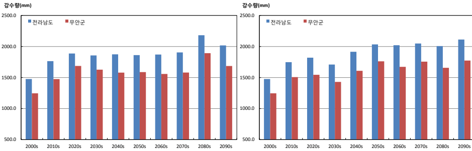
그림 3-4. 전라남도과 무안군의 연강수량(mm) 시계열 (RCP4.5(좌), RCP8.5(우))
