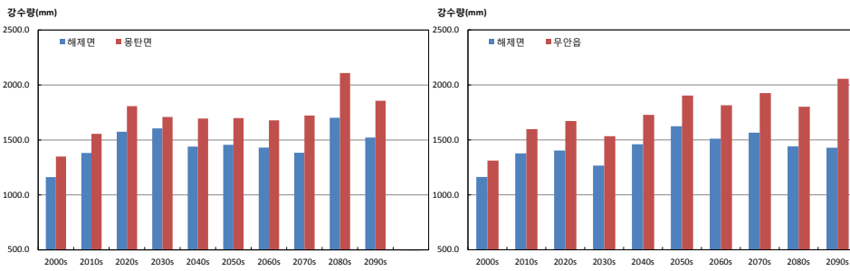
그림 3-5. 연강수량(mm) 증가율이 가장 큰 지역 (몽탄면, 무안읍)과 작은 지역(해제면)의 시계열 (RCP4.5(좌), RCP8.5(우))
