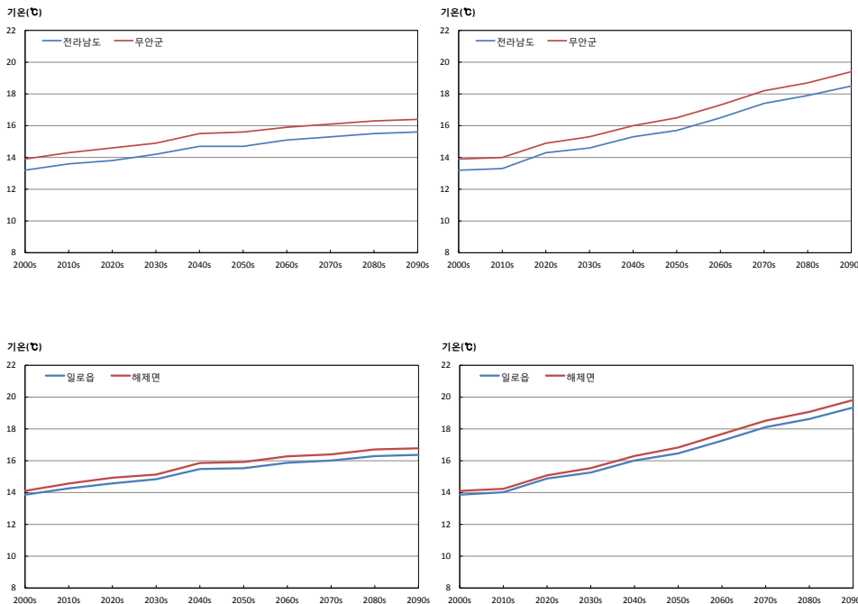
그림 3-1. 전라남도과 무안군의 평균기온(℃) 시계열(RCP4.5(좌), RCP8.5(우))
