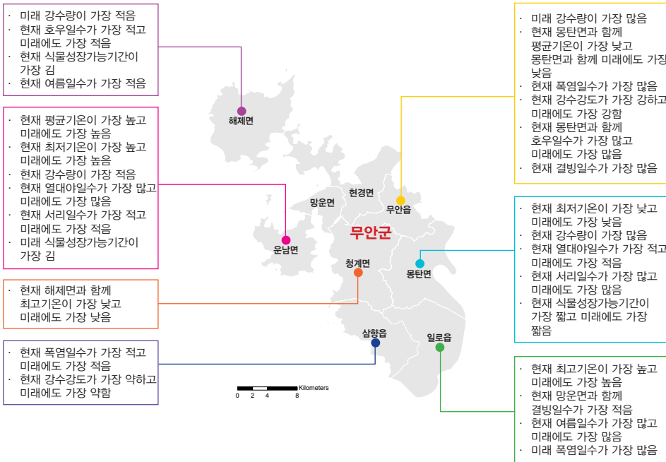
그림 5-1. 전라남도 무안군의 읍면별 기후변화 전망 요약
