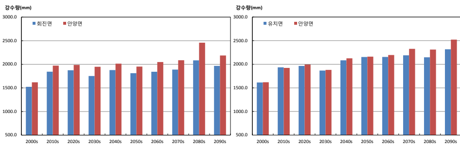
그림 3-5. 연강수량(mm) 증가율이 가장 큰 지역 (안양면)과 작은 지역(회진면, 유치면)의 시계열 (RCP4.5(좌), RCP8.5(우))
