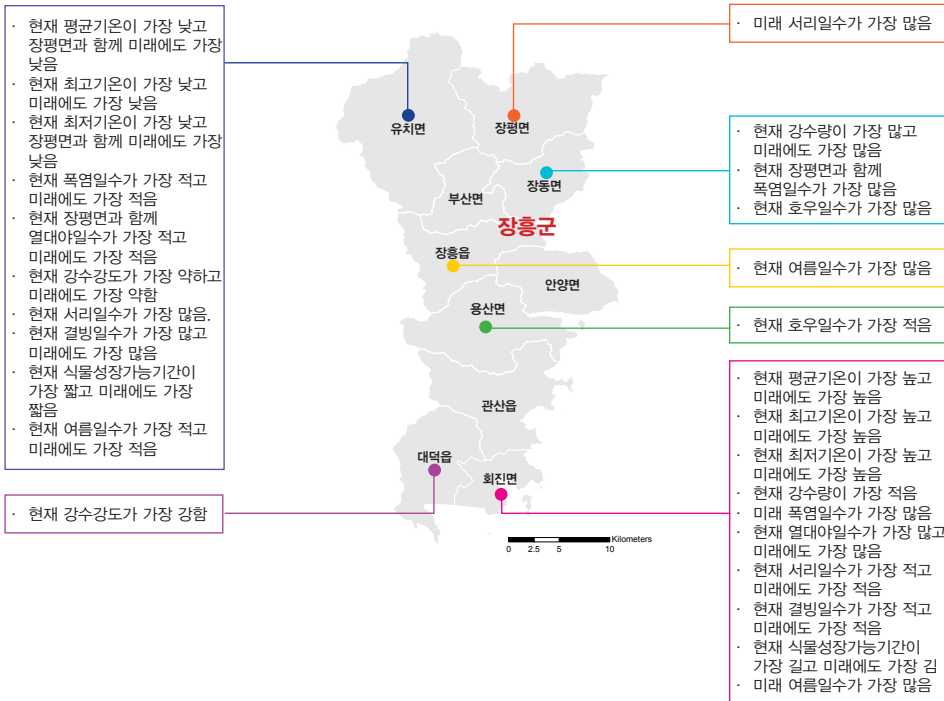
그림 5-1. 전라남도 장흥군의 읍면별 기후변화 전망 요약
