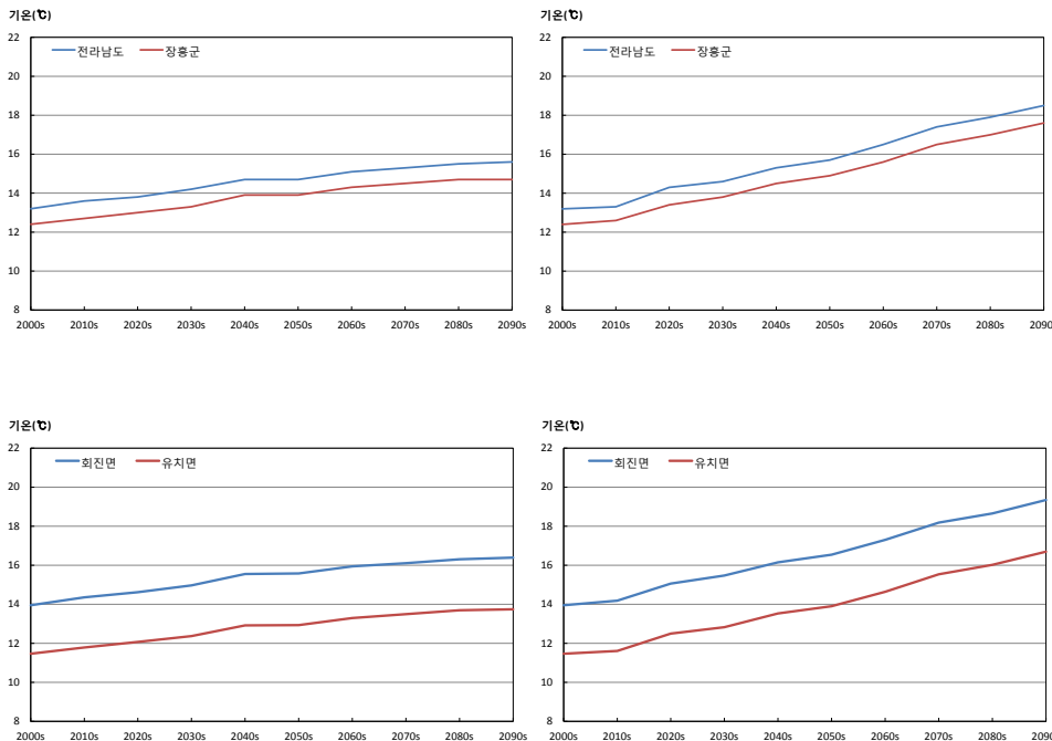
그림 3-1. 전라남도과 장흥군의 평균기온(℃) 시계열(RCP4.5(좌), RCP8.5(우))
