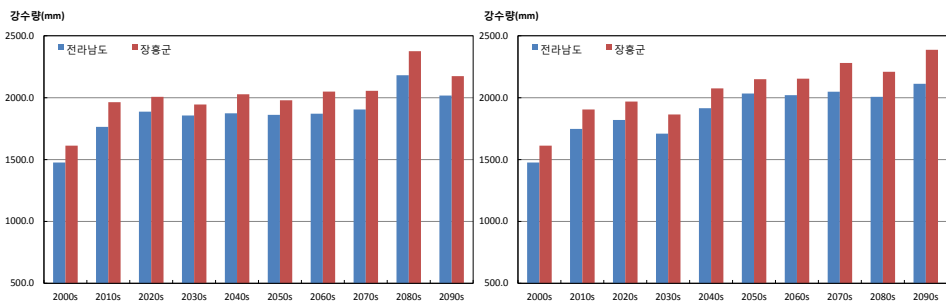
그림 3-4. 전라남도과 장흥군의 연강수량(mm) 시계열 (RCP4.5(좌), RCP8.5(우))
