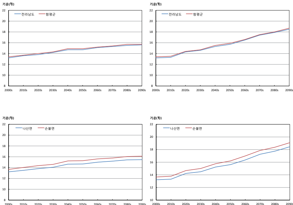
그림 3-1. 전라남도과 함평군의 평균기온(℃) 시계열(RCP4.5(좌), RCP8.5(우))
