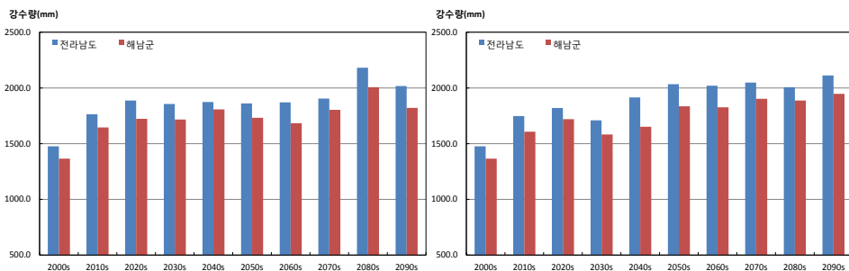
그림 3-4. 전라남도과 해남군의 연강수량(mm) 시계열 (RCP4.5(좌), RCP8.5(우))
