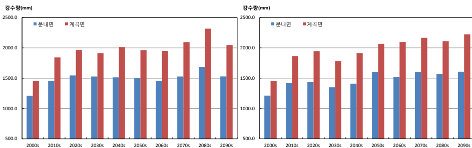
그림 3-5. 연강수량(mm) 증가율이 가장 큰 지역 (계곡면)과 작은 지역(문내면)의 시계열 (RCP4.5(좌), RCP8.5(우))
