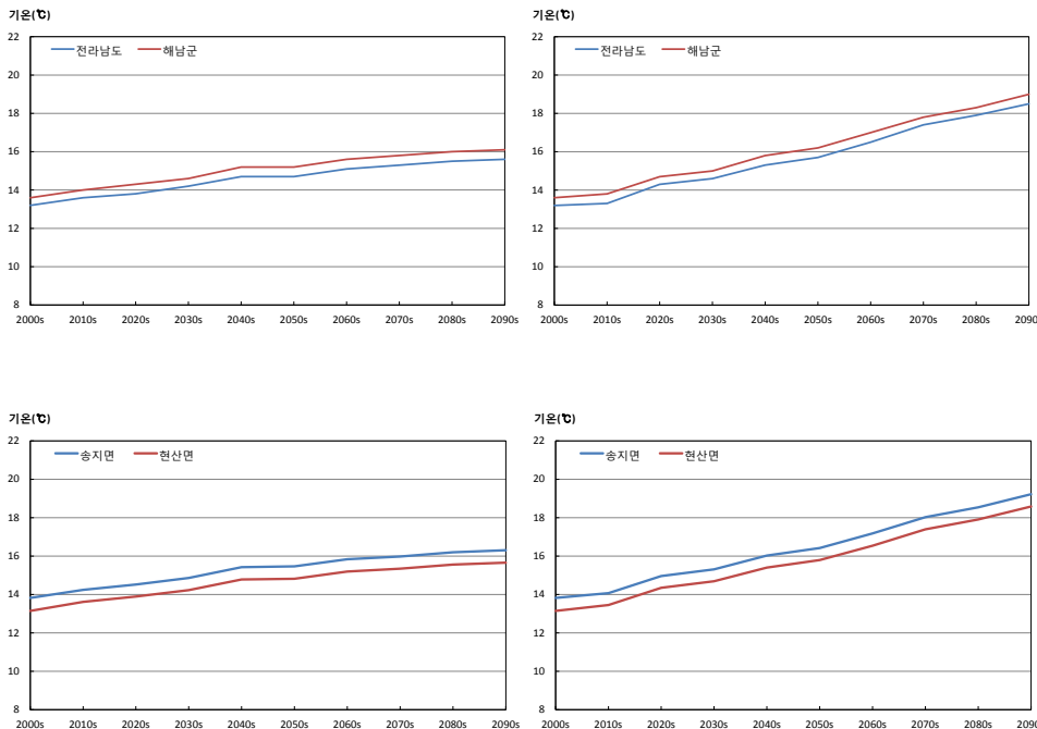
그림 3-1. 전라남도과 해남군의 평균기온(℃) 시계열(RCP4.5(좌), RCP8.5(우))
