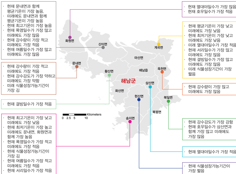
그림 5-1. 전라남도 해남군의 읍면별 기후변화 전망 요약
