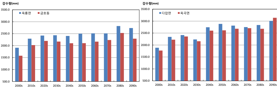
그림 3-5. 연강수량(mm) 증가율이 가장 큰 지역 (금호동, 옥곡면)과 작은 지역(옥룡면, 다압면)의 시계열(RCP4.5(좌), RCP8.5(우))
