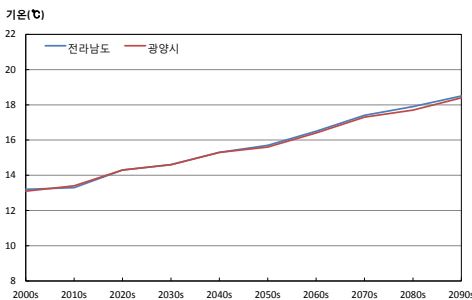
그림 3-1. 전라남도과 광양시의 평균기온(°C) 시계열(RCP4.5(좌), RCP8.5(우))
