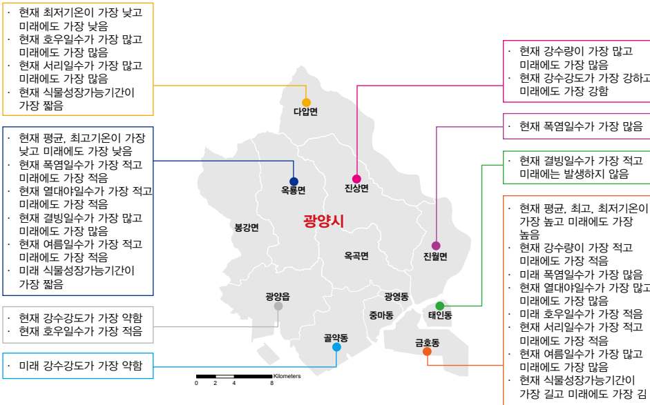
그림 5-1. 전라남도 광양시의 읍면동별 기후변화 전망 요약(RCP8.5 2071~2100년)
