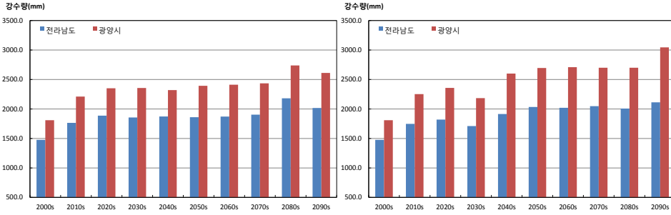
그림 3-4. 전라남도과 광양시의 연강수량(mm) 시계열 (RCP4.5(좌), RCP8.5(우))
