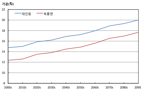
그림 3-2. 평균기온(°C) 증가율이 가장 큰 지역 (봉강면, 옥룡면)과 작은 지역(태인동)의 시계열(RCP4.5(좌), RCP8.5(우))
