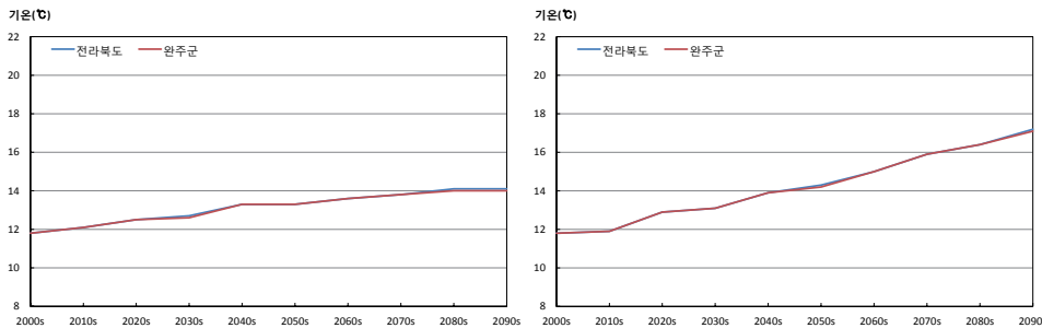
그림 3-1. 전라북도와 완주군의 평균기온(℃) 시계열(RCP4.5(좌), RCP8.5(우))
