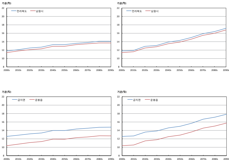
그림 3-1. 전라북도와 남원시의 평균기온(℃) 시계열(RCP4.5(좌), RCP8.5(우))
