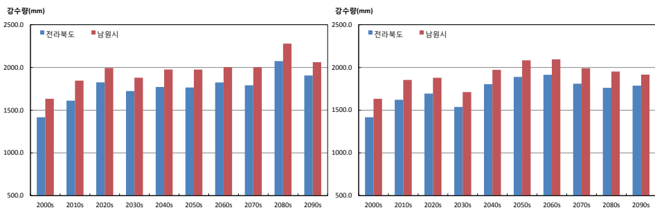
그림 3-4. 전라북도와 남원시의 연강수량(mm) 시계열 (RCP4.5(좌), RCP8.5(우))
