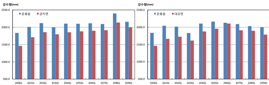
그림 3-5. 연강수량(mm) 증가율이 가장 큰 지역 (금지면, 대강면)과 작은 지역(운봉읍)의 시계열 (RCP4.5(좌), RCP8.5(우))
