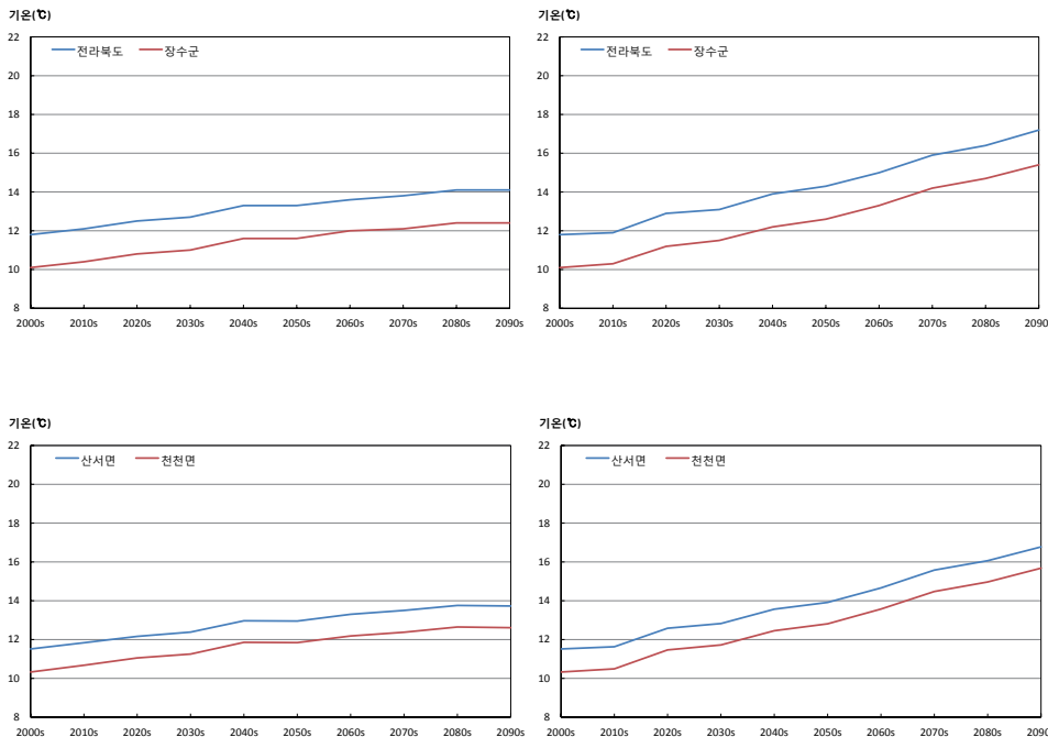
그림 3-1. 전라북도와 장수군의 평균기온(℃) 시계열(RCP4.5(좌), RCP8.5(우))
