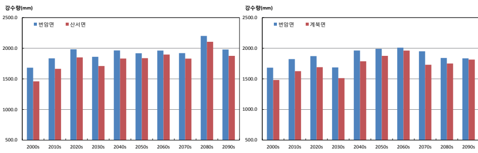
그림 3-5. 연강수량(mm) 증가율이 가장 큰 지역 (산서면, 계북면)과 작은 지역(빈암면)의 시계열 (RCP4.5(좌), RCP8.5(우))
