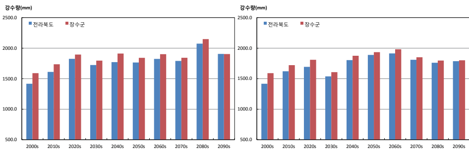
그림 3-4. 전라북도과 장수군의 연강수량(mm) 시계열 (RCP4.5(좌), RCP8.5(우))
