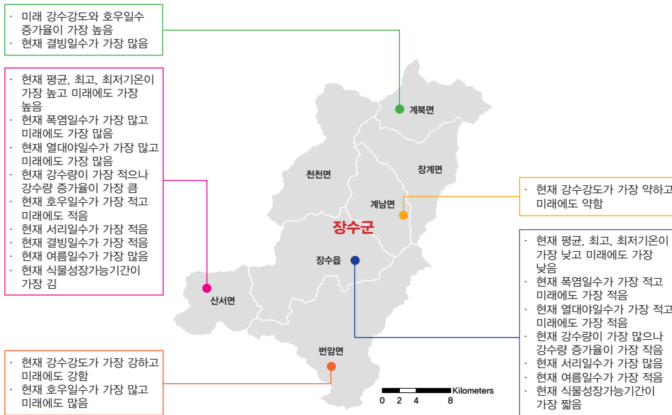
그림 5-1. 전라북도 장수군의 읍면별 기후변화 전망 요약
