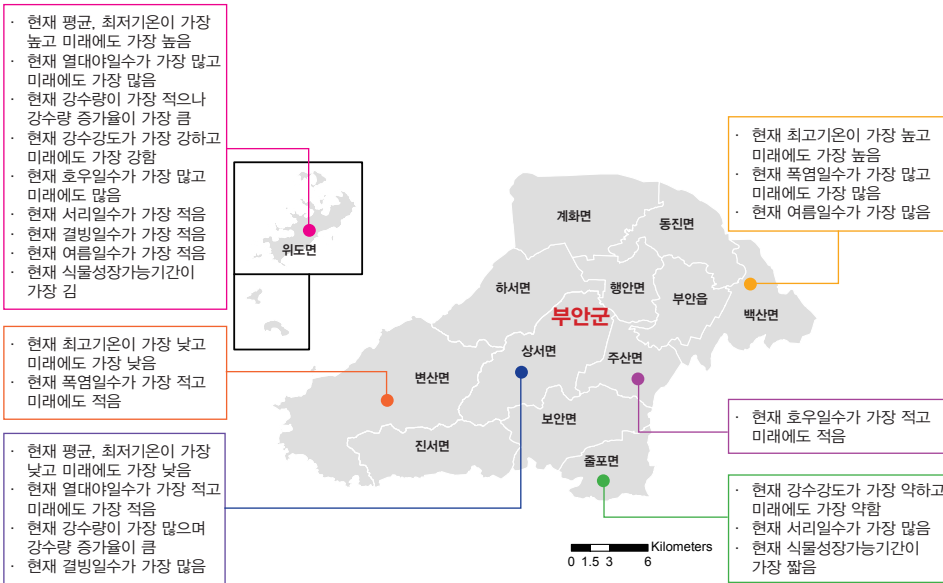
그림 5-1. 전라북도 부안군의 읍면별 기후변화 전망 요약
