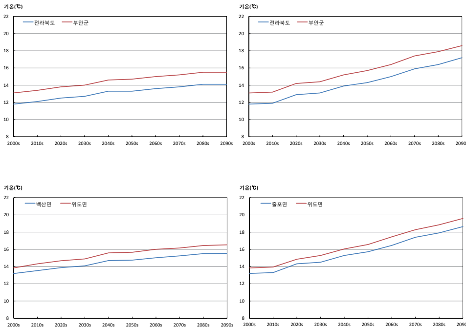
그림 3-1. 전라북도와 부안군의 평균기온(℃) 시계열(RCP4.5(좌), RCP8.5(우))
