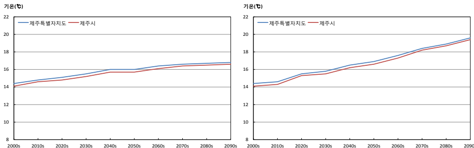
그림 3-1. 제주특별자치도와 제주시의 평균기온(℃) 시계열(RCP4.5(좌), RCP8.5(우))
