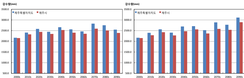
그림 3-4. 제주특별자치도와 제주시의 연강수량(mm) 시계열 (RCP4.5(좌), RCP8.5(우))
