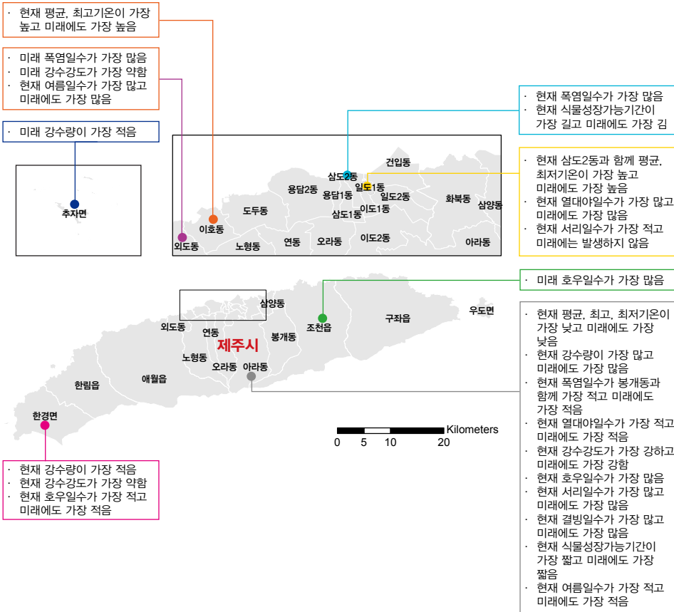
그림 5-1. 제주특별자치도 제주시의 읍면동별 기후변화 전망 요약(RCP8.5 2071~2100년)
