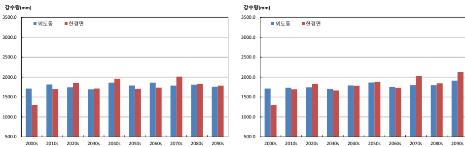
그림 3-5. 연강수량(mm) 증가율이 가장 큰 지역 (한경면)과 작은 지역(외도동)의 시계열 (RCP4.5(좌), RCP8.5(우))
