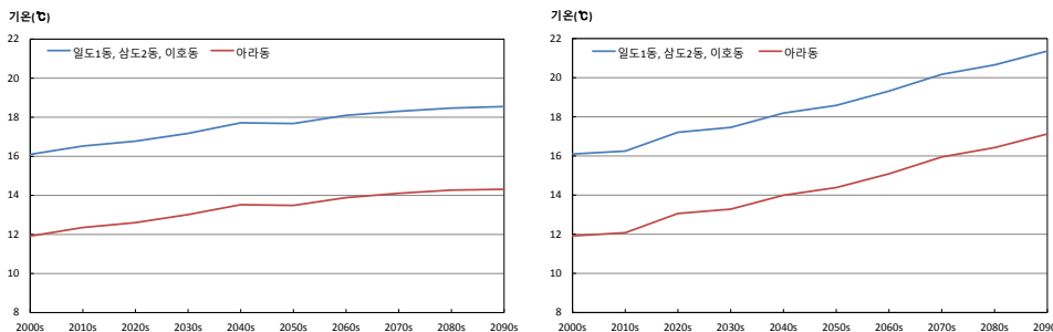
그림 3-2. 평균기온(℃) 증가율이 가장 큰 지역(아라동)과 작은 지역(일도1동, 삼도2동, 이호동)의 시계열(RCP4.5(좌), RCP8.5(우))
