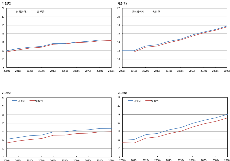
그림 3-1. 인천광역시와 웅진군의 평균기온(℃) 시계열(RCP4.5(좌), RCP8.5(우))
