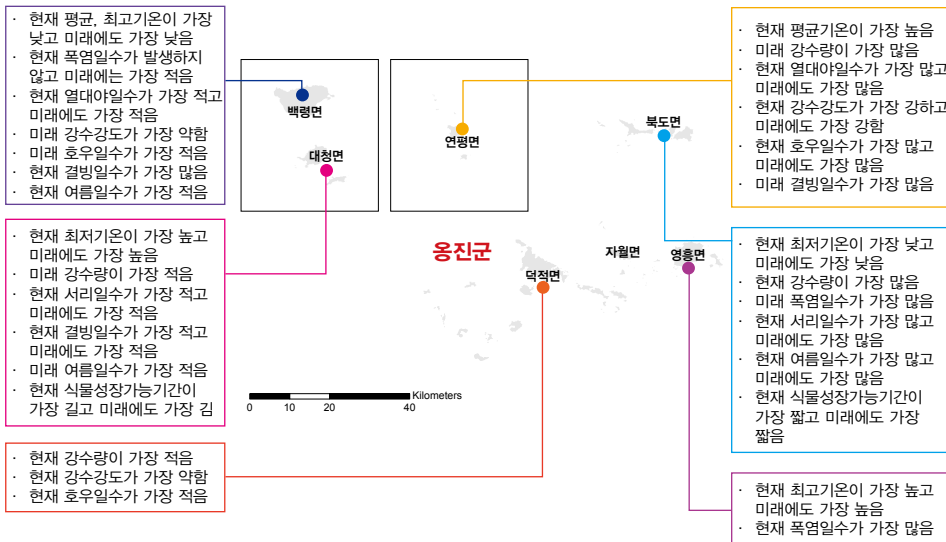
그림 5-1. 인천광역시 옹진군의 면별 기후변화 전망 요약(RCP8.5 2071~2100년)
