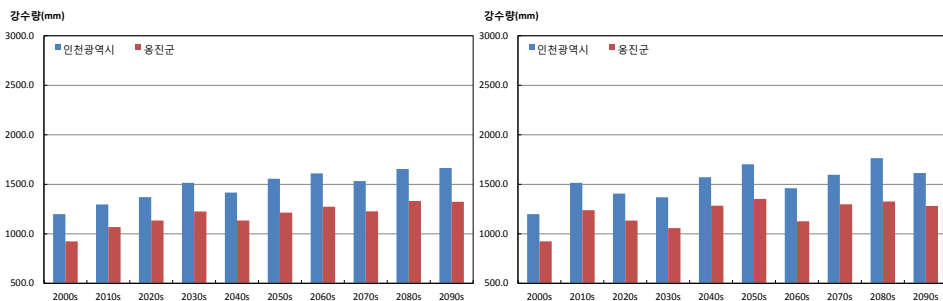
그림 3-4. 인천광역시와 영진군의 연강수량(mm) 시계열 (RCP4.5(좌), RCP8.5(우))
