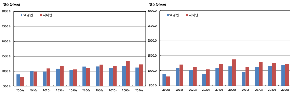
그림 3-5. 연강수량(mm) 증가율이 가장 큰 지역(덕적면)과 작은 지역(백령면)의 시계열(RCP4.5(좌), RCP8.5(우))
