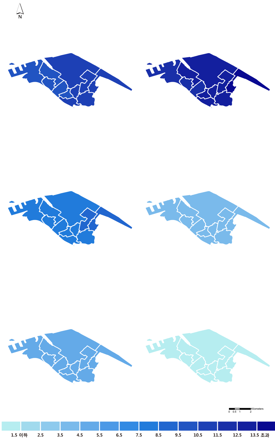
그림 3-11. 동구의 동별 결빙일수(일) 분포도 (RCP4.5(좌)/8.5(우), 2011~2040년(상), 2041~2070년(중), 2071~2100년(하))
