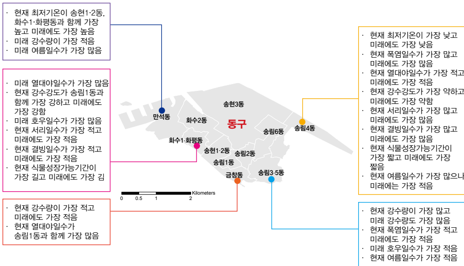
그림 5-1. 인천광역시 동구의 동별 기후변화 전망 요약(RCP8.5 2071~2100년)
