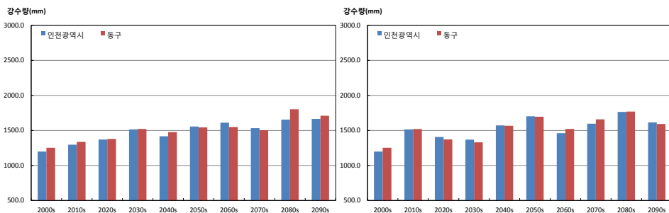
그림 3-4. 인천광역시와 동구의 연강수량(mm) 시계열 (RCP4.5(좌), RCP8.5(우))
