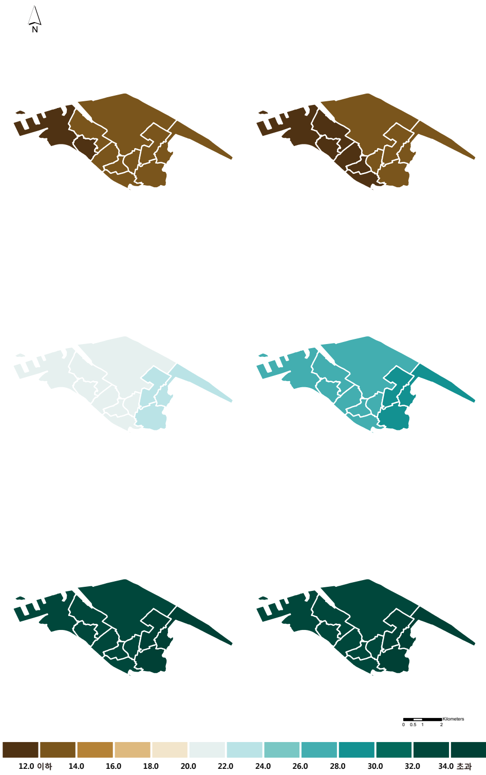
그림 3-7. 동구의 동별 강수량 증가율(%) (2001~2010년 대비) 분포도 (RCP4.5(좌)/8.5(우), 2011~2040년(상), 2041~2070년(중), 2071~2100년(하))
