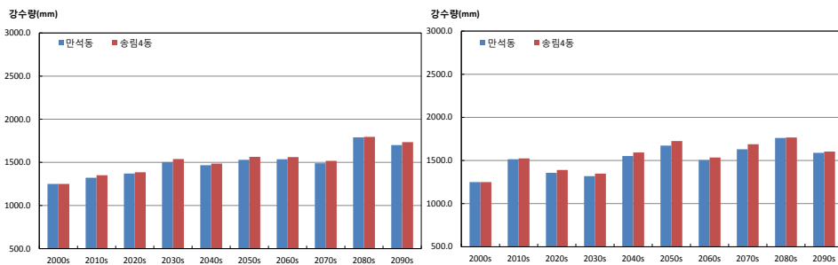
그림 3-5. 연강수량(mm) 증가율이 가장 큰 지역 (송림4동)과 작은 지역(만석동)의 시계열(RCP4.5(좌), RCP8.5(우))
