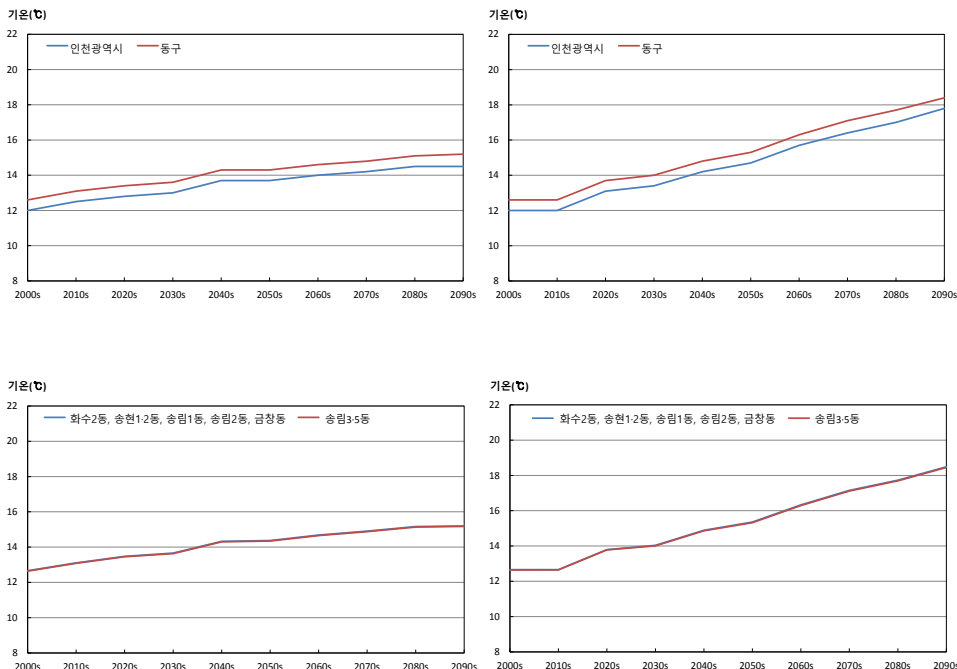
그림 3-1. 인천광역시와 동구의 평균기온(°C) 시계열(RCP4.5(좌), RCP8.5(우))
