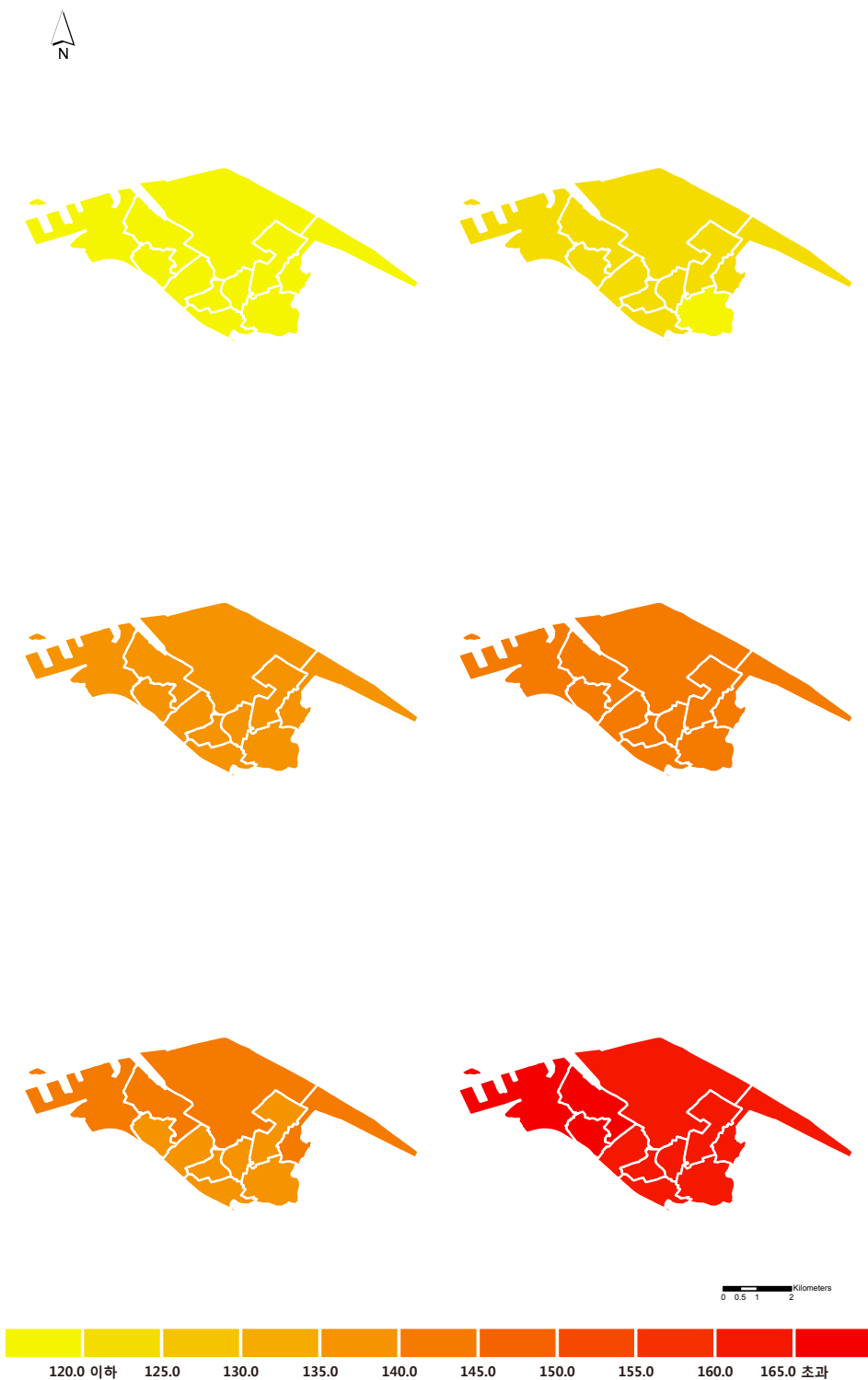
그림 3-13. 동구의 동별 여름일수(일) 분포도 (RCP4.5(좌)/8.5(우), 2011~2040년(상), 2041~2070년(중), 2071~2100년(하))
