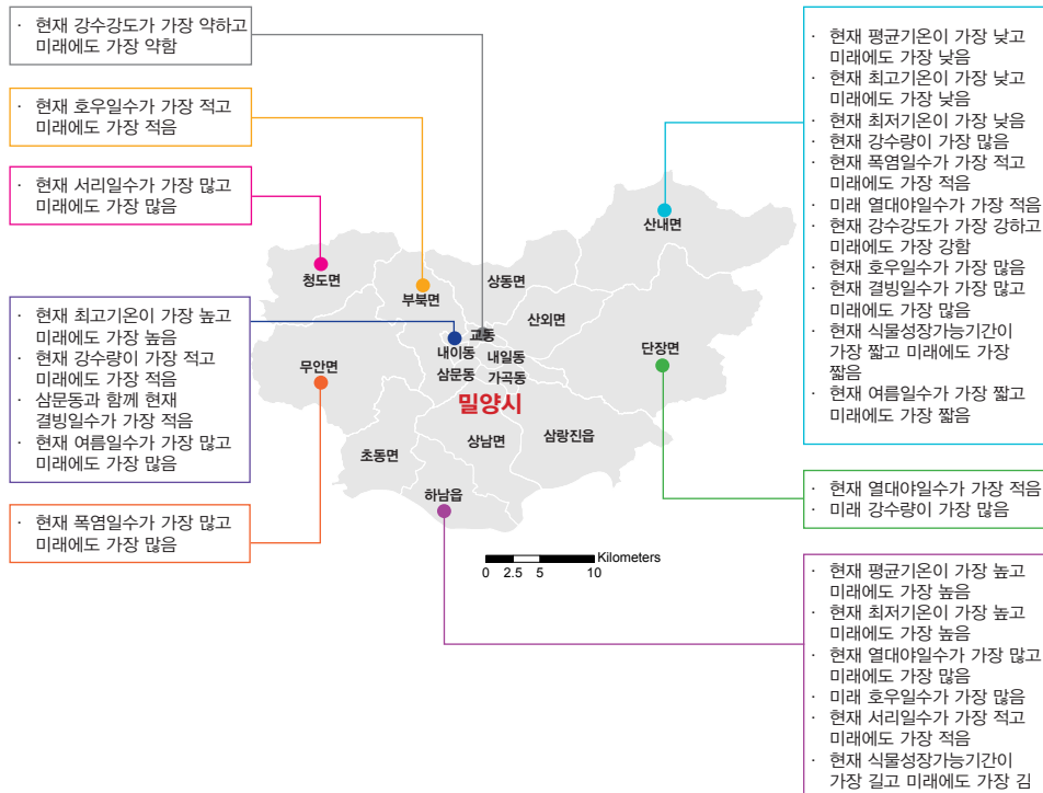
그림 5-1. 경상남도 밀양시의 읍면동별 기후변화 전망 요약
