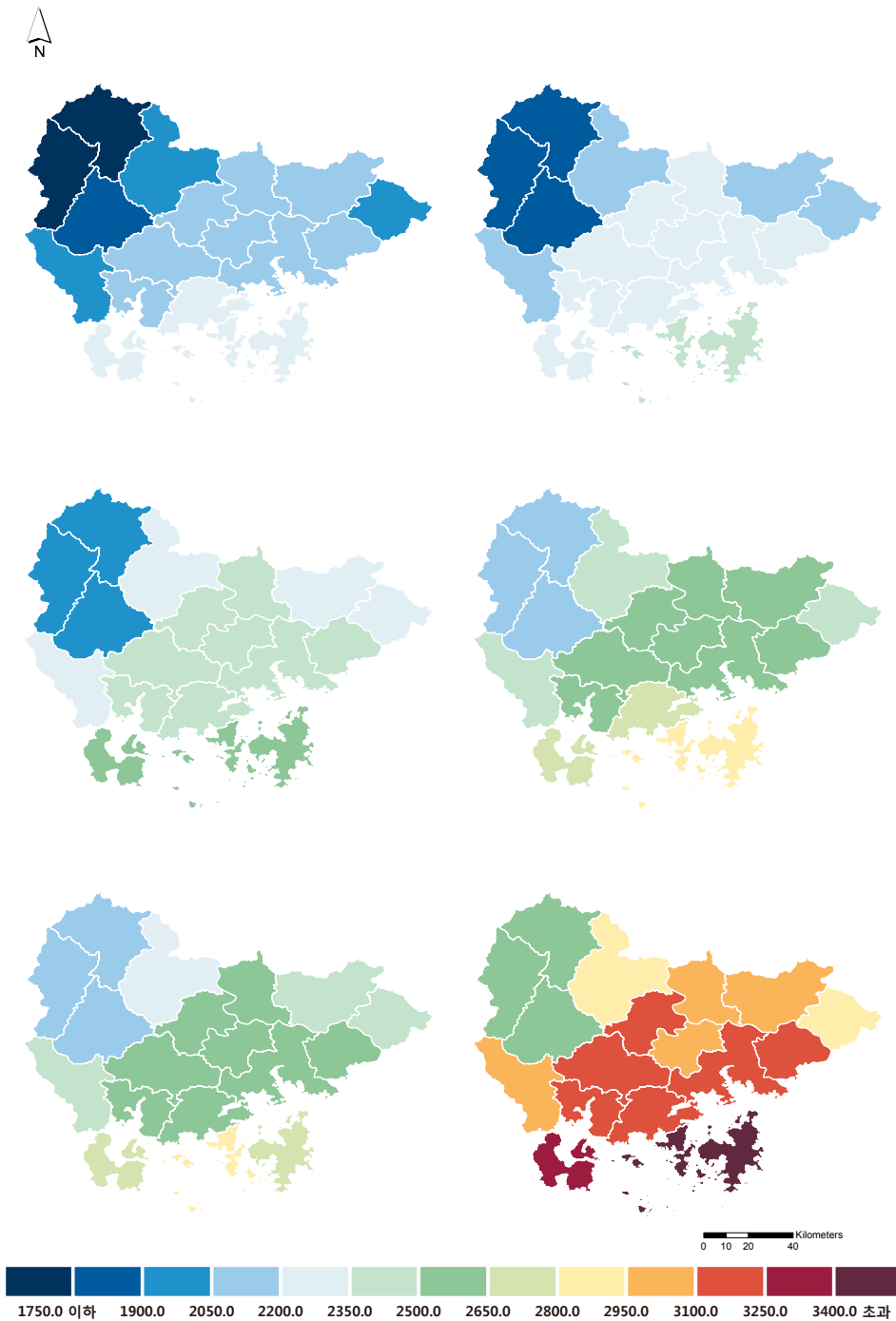
그림 4-2. 경상남도 시군별 유효적산온도(10°C)(°C) 분포도 (RCP4.5(좌)/8.5(우), 2011~2040년(상), 2041~2070년(중), 2071~2100년(하))
