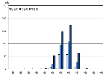
그림 4-5. 밀양시의 월별 냉방도일(도일)전망 (RCP4.5(좌), RCP8.5(우))
