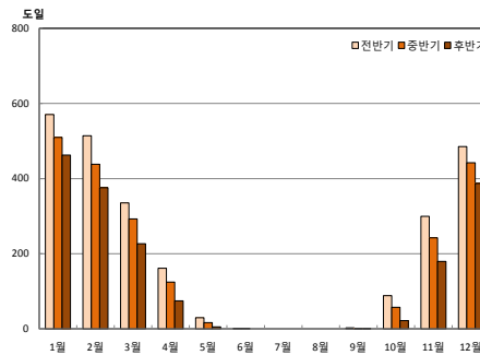
그림 4-6. 밀양시의 월별 난방도일(도일) 전망 (RCP4.5(좌), RCP8.5(우))
