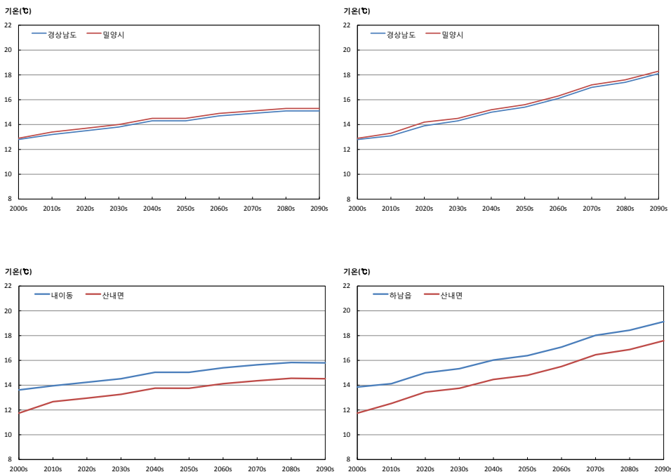
그림 3-1. 경상남도과 밀양시의 평균기온(℃) 시계열(RCP4.5(좌), RCP8.5(우))
