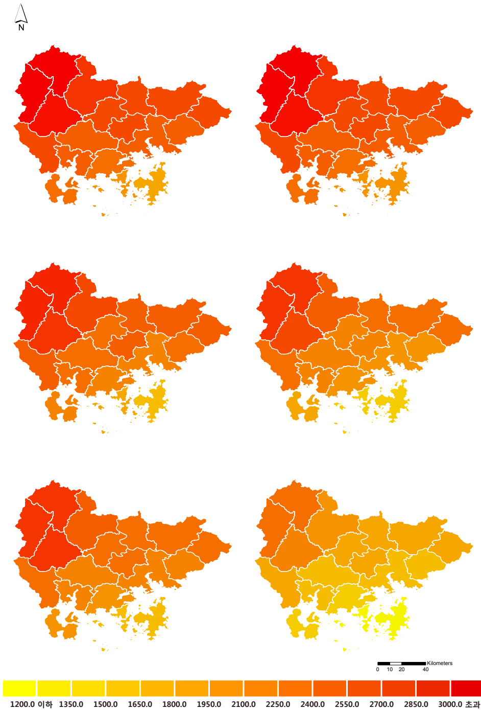
그림 4-8. 경상남도 시군별 난방도일(도일) 분포도 (RCP4.5(좌)/8.5(우), 2011~2040년(상), 2041~2070년(중), 2071~2100년(하))
