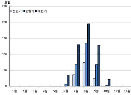
그림 4-5. 거제시의 월별 냉방도일(도일)전망 (RCP4.5(좌), RCP8.5(우))
