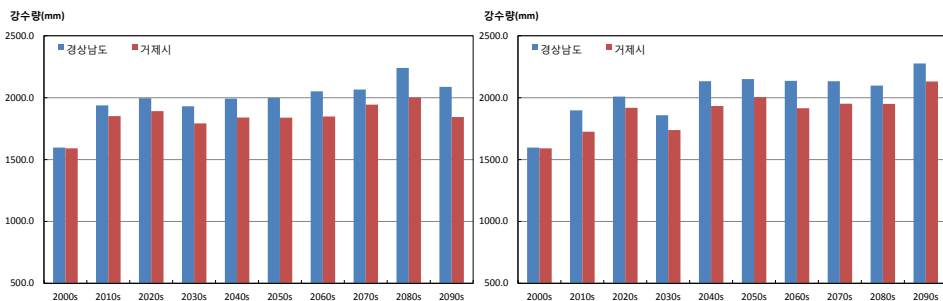
그림 3-4. 경상남도과 거제시의 연강수량(mm) 시계열 (RCP4.5(좌), RCP8.5(우))
