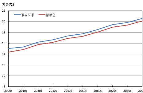
그림 3-2. 평균기온(℃) 증가율이 가장 큰 지역(남부면)과 작은 지역(장승포동)의 시계열(RCP4.5(좌), RCP8.5(우))
