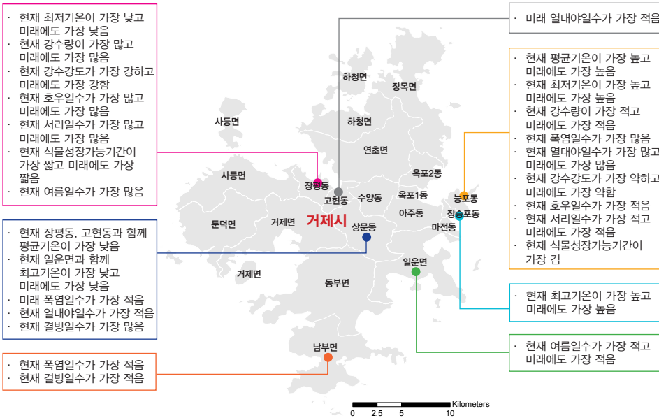
그림 5-1. 경상남도 거제시의 면동별 기후변화 전망 요약
