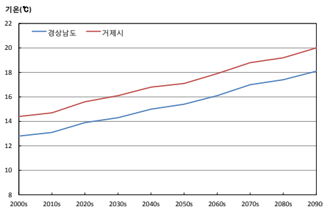
그림 3-1. 경상남도과 거제시의 평균기온(℃) 시계열(RCP4.5(좌), RCP8.5(우))
