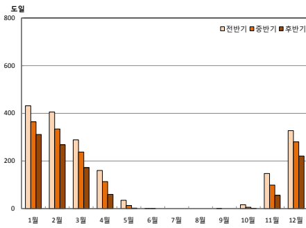
그림 4-6. 거제시의 월별 난방도일(도일) 전망 (RCP4.5(좌), RCP8.5(우))
