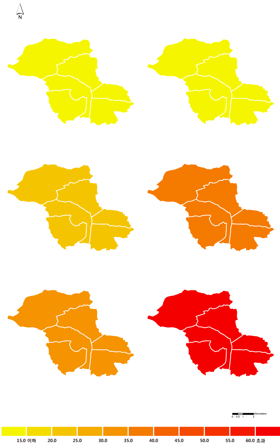
그림 3-9. 오산시의 동별 열대야일수(일) 분포도 (RCP4.5(좌)/8.5(우), 2011~2040년(상), 2041~2070년(중), 2071~2100년(하))
