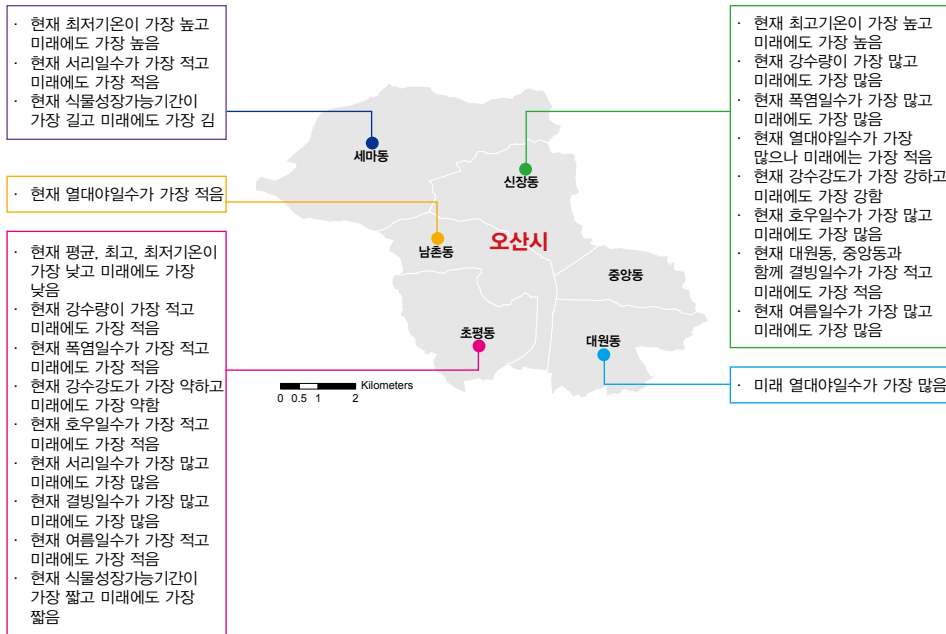
그림 5-1. 경기도 오산시의 동별 기후변화 전망 요약(RCP8.5 2071~2100년)
