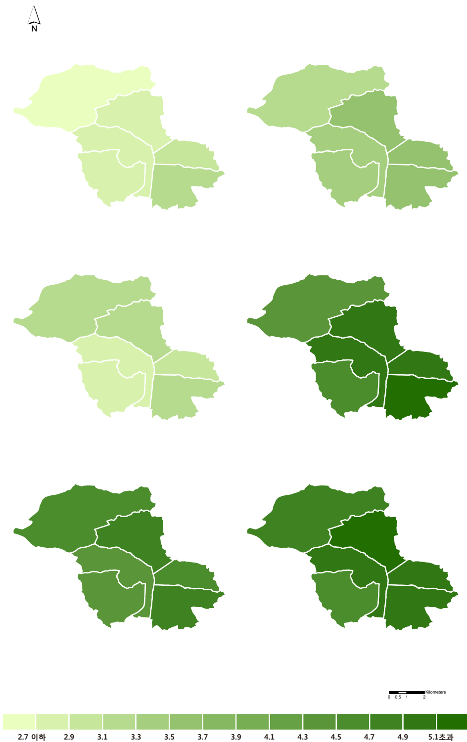
그림 3-15. 오산시의 동별 호우일수(일) 분포도 (RCP4.5(좌)/8.5(우), 2011~2040년(상), 2041~2070년(중), 2071~2100년(하))
