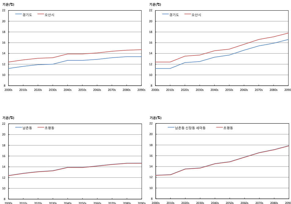
그림 3-1. 경기도와 오산시의 평균기온(℃) 시계열(RCP4.5(좌), RCP8.5(우))
