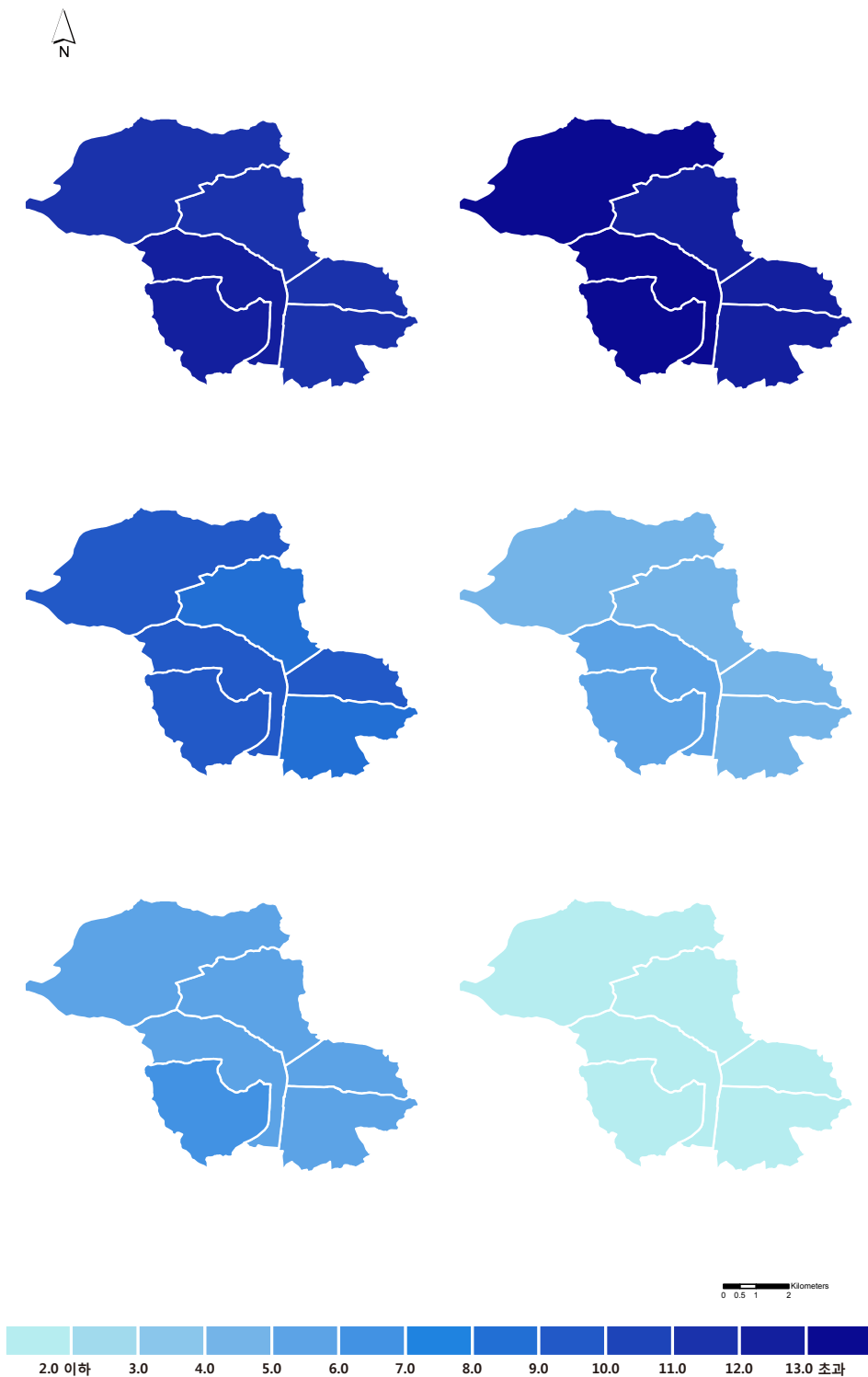
그림 3-11. 오산시의 동별 결빙일수(일) 분포도 (RCP4.5(좌)/8.5(우), 2011~2040년(상), 2041~2070년(중), 2071~2100년(하))
