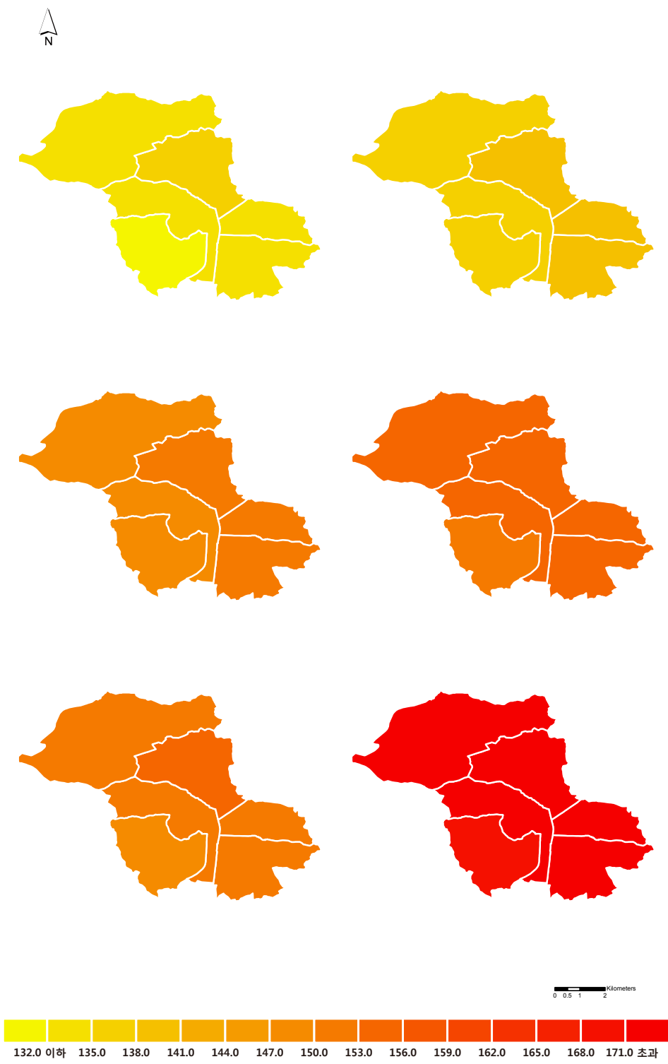
그림 3-13. 오산시의 동별 여름일수(일) 분포도 (RCP4.5(좌)/8.5(우), 2011~2040년(상), 2041~2070년(중), 2071~2100년(하))
