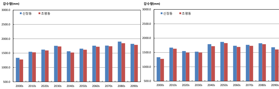
그림 3-5. 연강수량(mm) 증가율이 가장 큰 지역 (조평동)과 작은 지역(신장동)의 시계열(RCP4.5(좌), RCP8.5(우))
