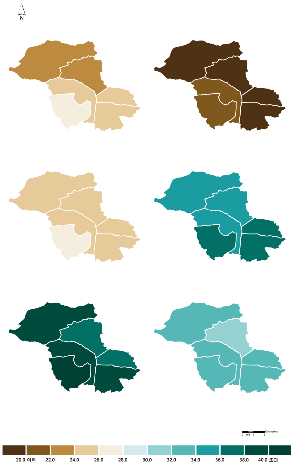
그림 3-7. 오산시의 동별 강수량 증가율(%) (2001~2010년 대비) 분포도 (RCP4.5(좌)/8.5(우), 2011~2040년(상), 2041~2070년(중), 2071~2100년(하))
