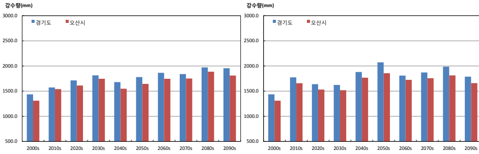
그림 3-4. 경기도와 오산시의 연강수량(mm) 시계열 (RCP4.5(좌), RCP8.5(우))
