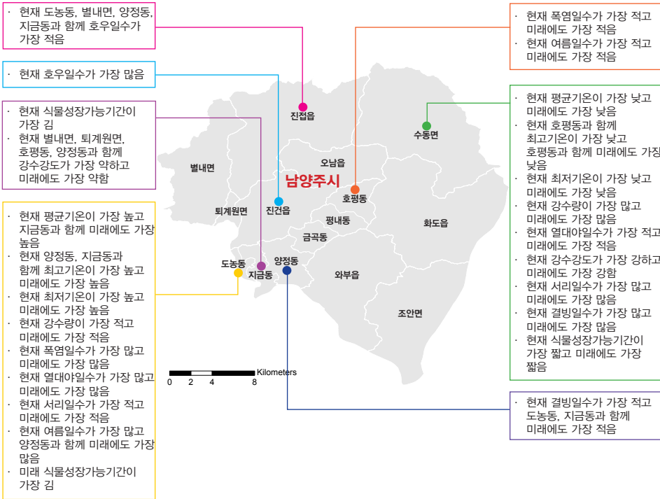
그림 5-1. 경기도 남양주시의 읍면동별 기후변화 전망 요약
