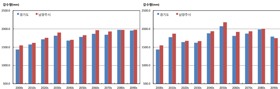
그림 3-4. 경기도와 남양주시의 연강수량(mm) 시계열 (RCP4.5(좌), RCP8.5(우))
