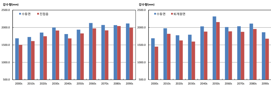
그림 3-5. 연강수량(mm) 증가율이 가장 큰 지역 (진접읍, 퇴계원면)과 작은 지역(수동면)의 시계열(RCP4.5(좌), RCP8.5(우))
