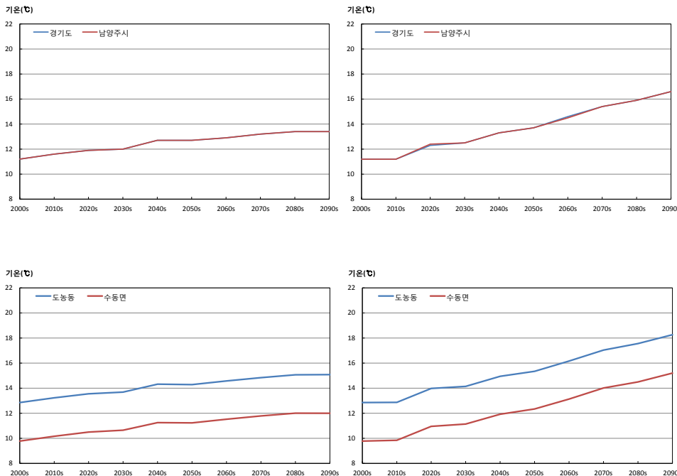
그림 3-1. 경기도와 남양주시의 평균기온(℃) 시계열(RCP4.5(좌), RCP8.5(우))
