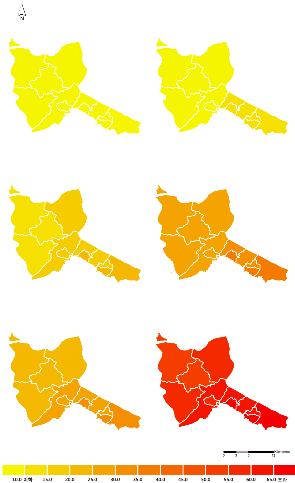
그림 3-9. 김포시의 읍면동별 열대야일수(일) 분포도 (RCP4.5(좌)/8.5(우), 2011~2040년(상), 2041~2070년(중), 2071~2100년(하))
