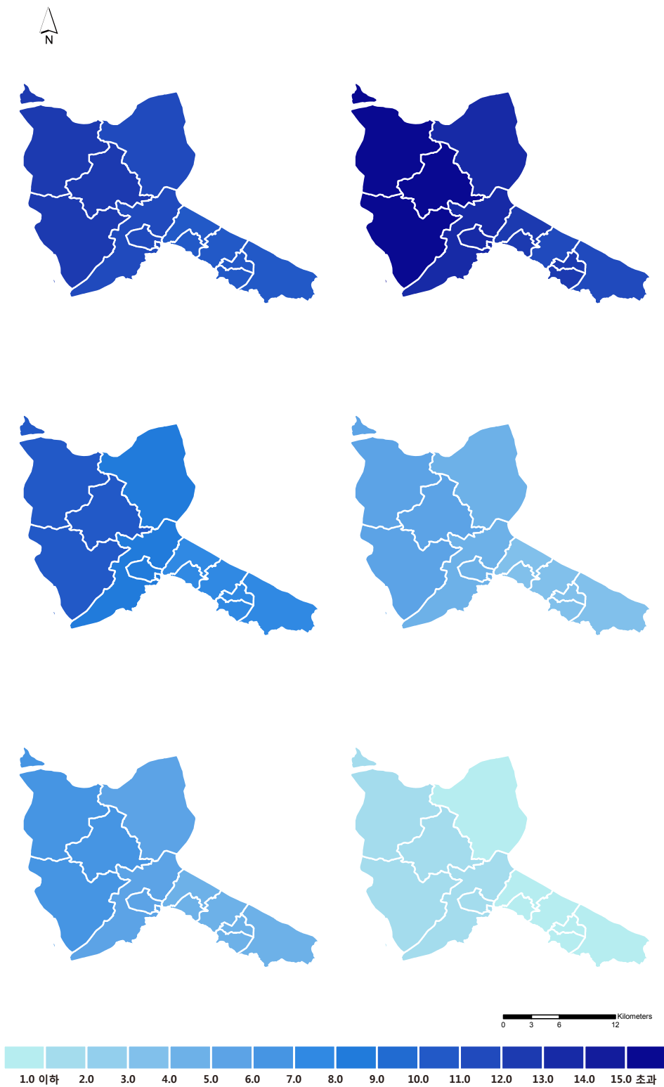
그림 3-11. 김포시의 읍면동별 결빙일수(일) 분포도 (RCP4.5(좌)/8.5(우), 2011~2040년(상), 2041~2070년(중), 2071~2100년(하))
