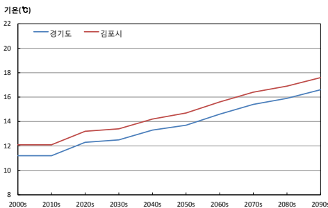
그림 3-1. 경기도와 김포시의 평균기온(℃) 시계열(RCP4.5(좌), RCP8.5(우))
