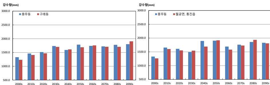
그림 3-5. 연강수량(mm) 증가율이 가장 큰 지역 (구래동, 월곶면, 통진읍)과 작은 지역(жом문동)의 시계열(RCP4.5(좌), RCP8.5(우))
