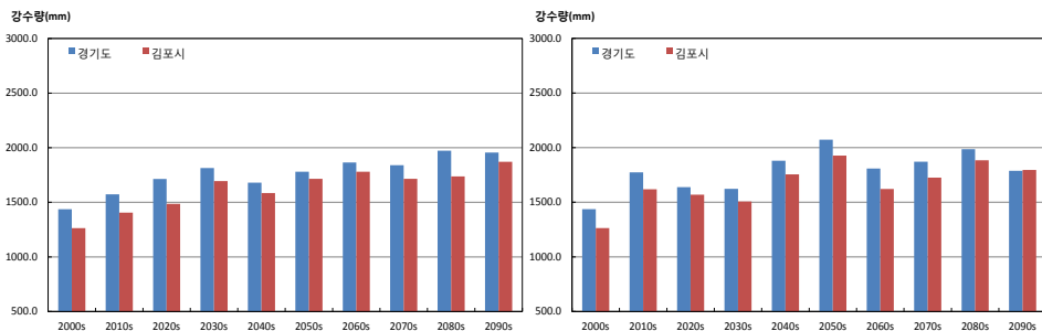
그림 3-4. 경기도와 김포시의 연강수량(mm) 시계열 (RCP4.5(좌), RCP8.5(우))
