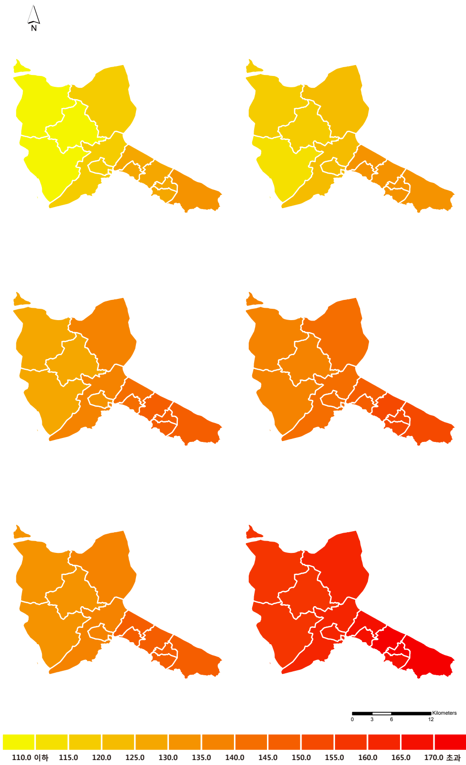
그림 3-13. 김포시의 읍면동별 여름일수(일) 분포도 (RCP4.5(좌)/8.5(우), 2011~2040년(상), 2041~2070년(중), 2071~2100년(하))
