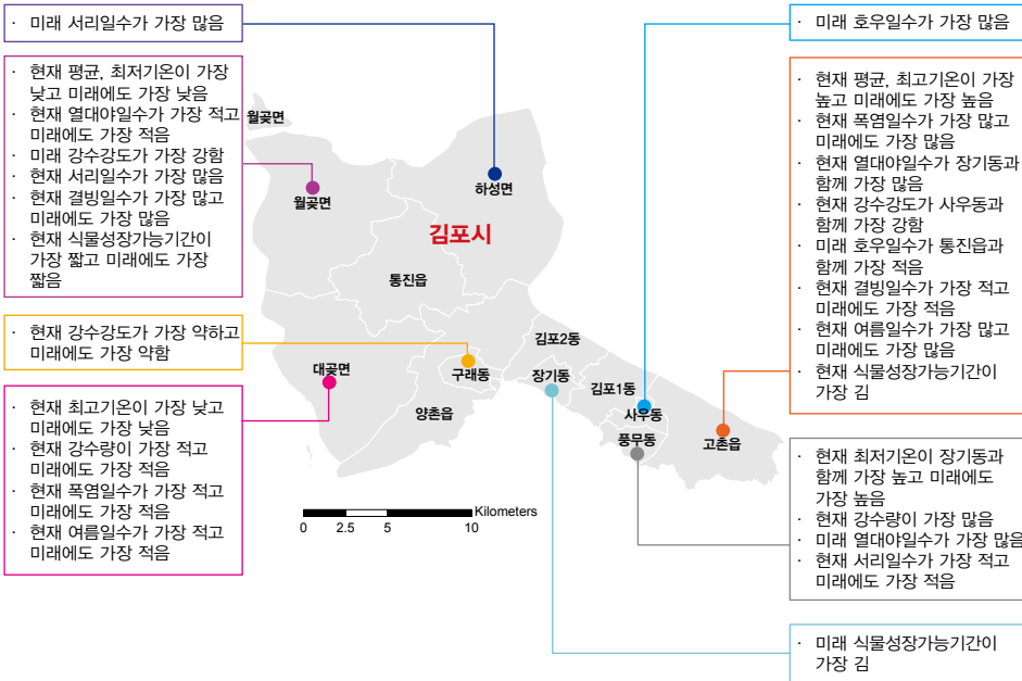
그림 5-1. 경기도 김포시의 읍면동별 기후변화 전망 요약(RCP8.5 2071~2100년)
