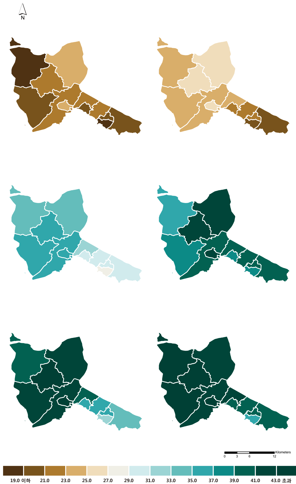
그림 3-7. 김포시의 읍면동별 강수량 증가율(%) (2001~2010년 대비) 분포도 (RCP4.5(좌)/8.5(우), 2011~2040년(상), 2041~2070년(중), 2071~2100년(하))
