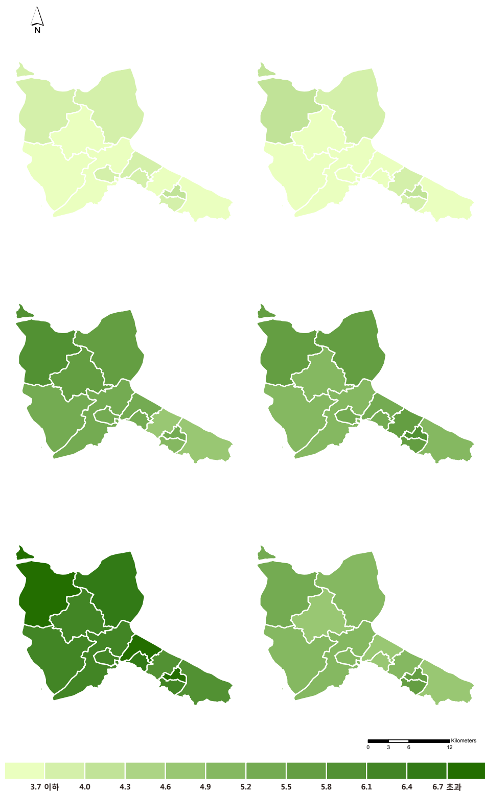
그림 3-15. 김포시의 읍면동별 호우일수(일) 분포도 (RCP4.5(좌)/8.5(우), 2011~2040년(상), 2041~2070년(중), 2071~2100년(하))
