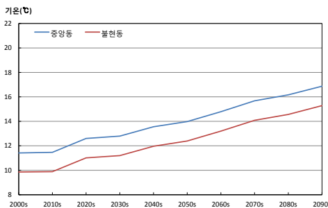
그림 3-2. 평균기온(℃) 증가율이 가장 큰 지역 (bulhyeondong)과 작은 지역(sangpaedong, jongsangdong)의 시계열(RCP4.5(좌), RCP8.5(우))
