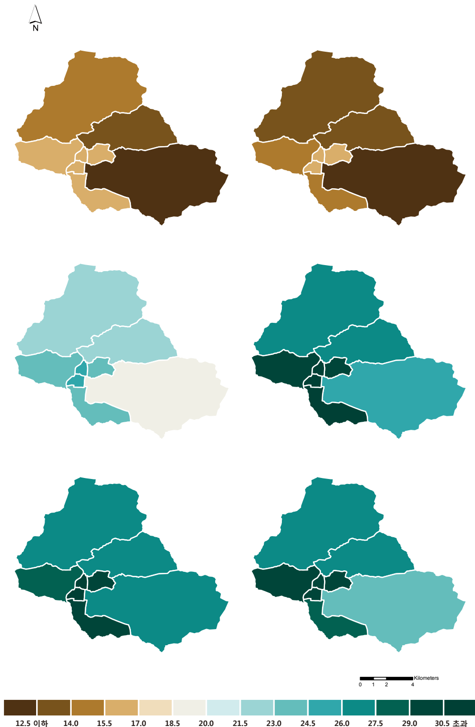
그림 3-7. 동두천시의 동별 강수량 증가율(%) (2001~2010년 대비) 분포도 (RCP4.5(좌)/8.5(우), 2011~2040년(상), 2041~2070년(중), 2071~2100년(하))
