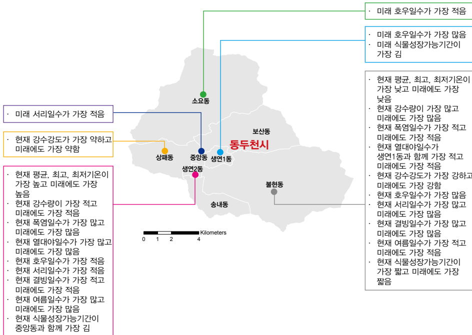
그림 5-1. 경기도 동두천시의 동별 기후변화 전망 요약(RCP8.5 2071~2100년)
