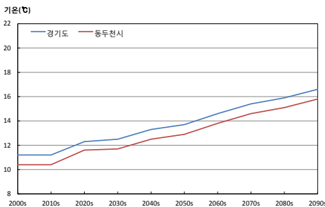
그림 3-1. 경기도와 동두천시의 평균기온(℃) 시계열(RCP4.5(좌), RCP8.5(우))
