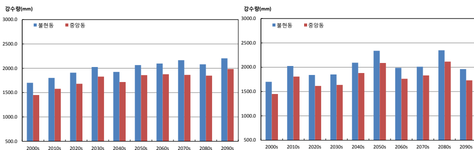
그림 3-5. 연강수량(mm) 증가율이 가장 큰 지역 (중앙동)과 작은 지역(불현동)의 시계열(RCP4.5(좌), RCP8.5(우))
