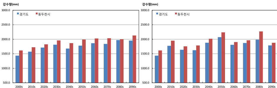
그림 3-4. 경기도와 동두천시의 연강수량(mm) 시계열 (RCP4.5(좌), RCP8.5(우))
