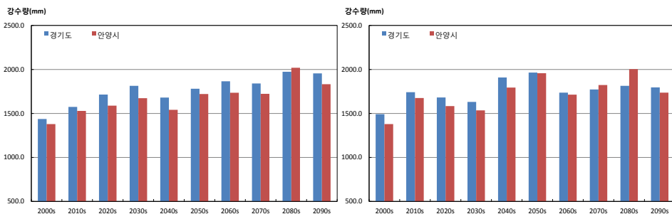
그림 3-4. 경기도와 안양시의 연강수량(mm) 시계열 (RCP4.5(좌), RCP8.5(우))
