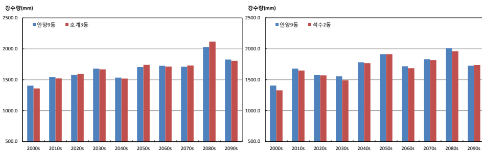
그림 3-5. 연강수량(mm) 증가율이 가장 큰 지역 (호계3동, 석수2동)과 작은 지역(안양9동)의 시계열 (RCP4.5(좌), RCP8.5(우))
