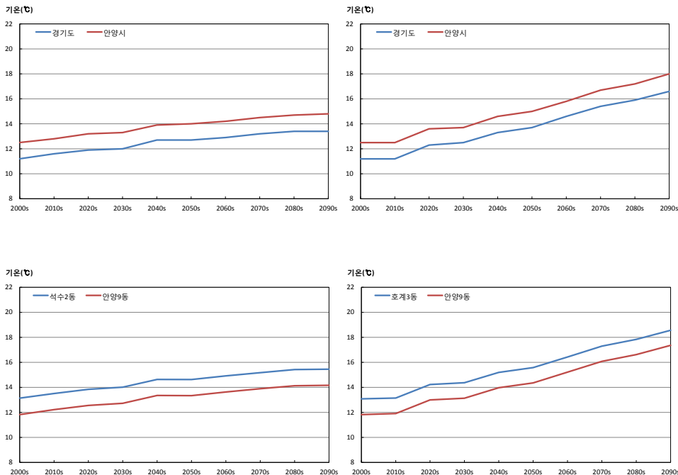
그림 3-1. 경기도와 안양시의 평균기온(℃) 시계열(RCP4.5(좌), RCP8.5(우))
