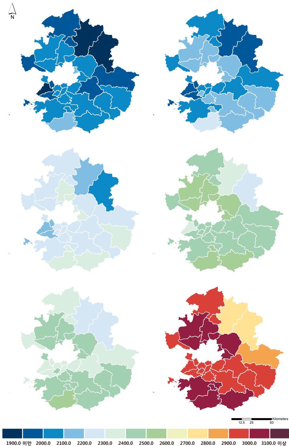
그림 4-2. 경기도 시군별 유효적산온도(10℃)(°C) 분포도 (RCP4.5(좌)/8.5(우), 2011~2040년(상), 2041~2070년(중), 2071~2100년(하))
