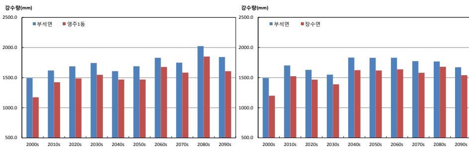
그림 3-5. 연강수량(mm) 증가율이 가장 큰 지역 (영주1동, 장수면)과 작은 지역(부석면)의 시계열 (RCP4.5(좌), RCP8.5(우))
