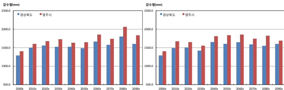
그림 3-4. 경상북도과 영주시의 연강수량(mm) 시계열 (RCP4.5(좌), RCP8.5(우))
