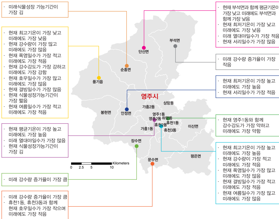
그림 5-1. 경상북도 영주시의 읍면동별 기후변화 전망 요약
