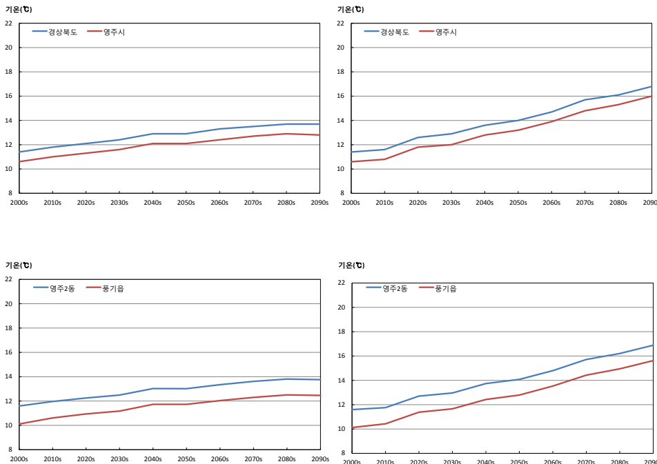
그림 3-1. 경상북도와 영주시의 평균기온(℃) 시계열(RCP4.5(좌), RCP8.5(우))
