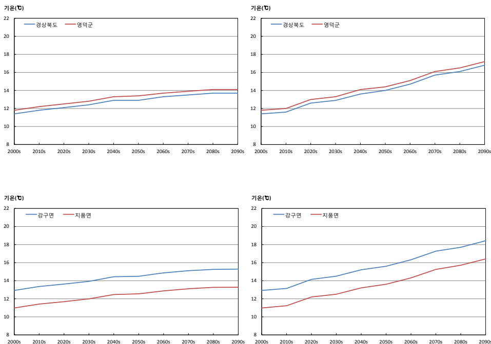
그림 3-1. 경상북도와 영덕군의 평균기온(℃) 시계열(RCP4.5(좌), RCP8.5(우))
