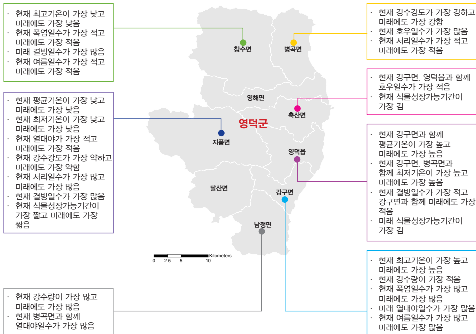
그림 5-1. 경상북도 영덕군의 읍면별 기후변화 전망 요약
