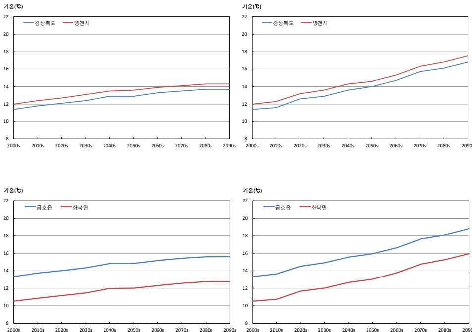
그림 3-1. 경상북도와 영천시의 평균기온(℃) 시계열(RCP4.5(좌), RCP8.5(우))
