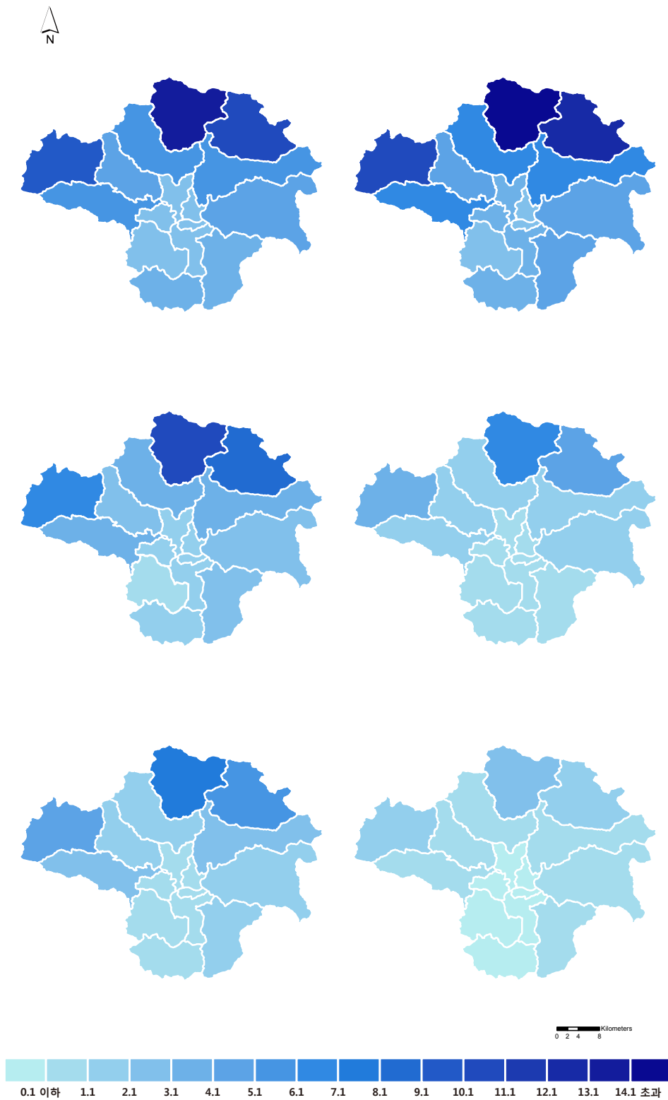
그림 3-11. 영천시 읍면동별 결빙일수(일) 분포도 (RCP4.5(좌)/8.5(우), 2011~2040년(상), 2041~2070년(중), 2071~2100년(하))
