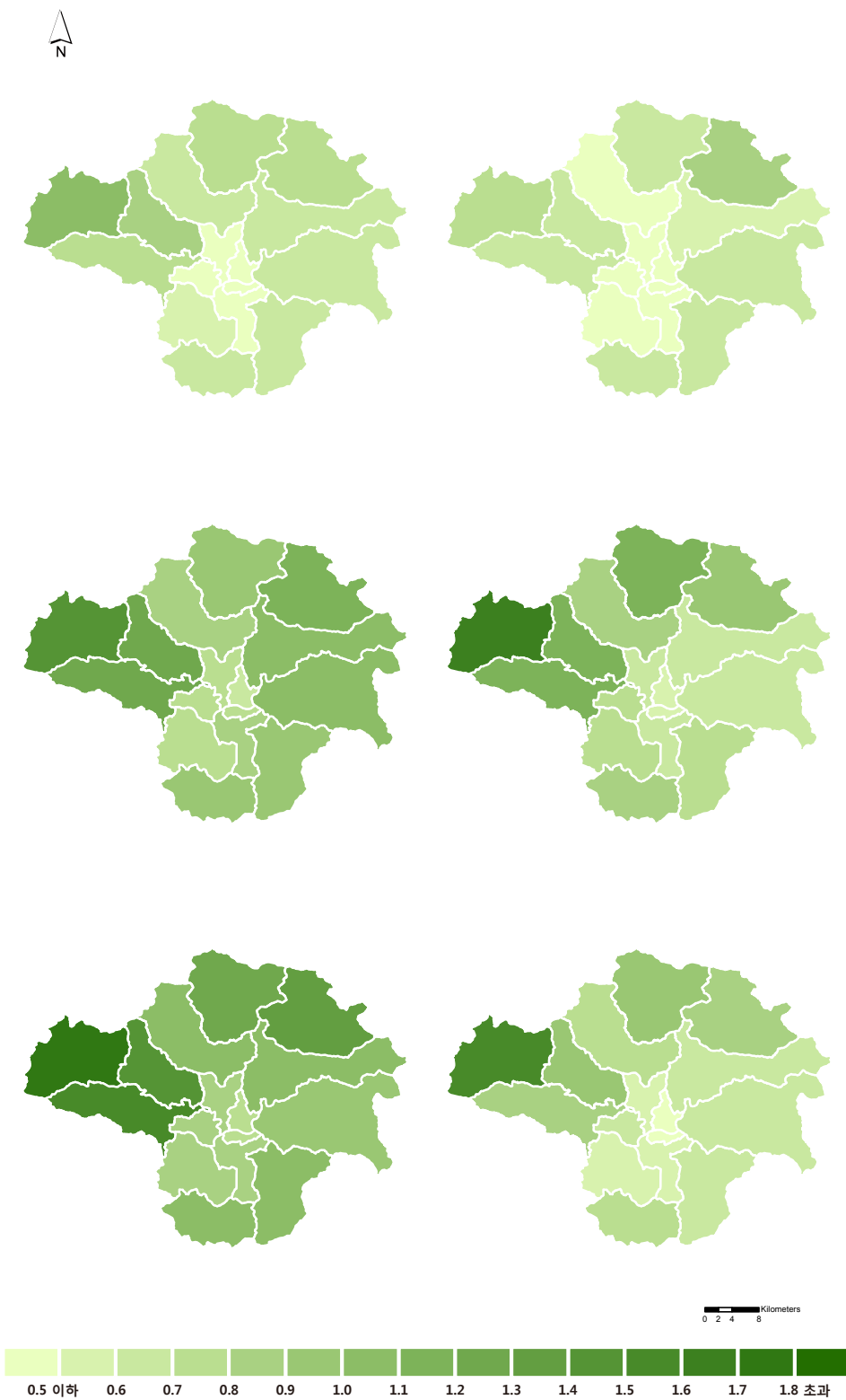
그림 3-15. 영천시의 읍면동별 호우일수(일) 분포도 (RCP4.5(좌)/8.5(우), 2011~2040년(상), 2041~2070년(중), 2071~2100년(하))
