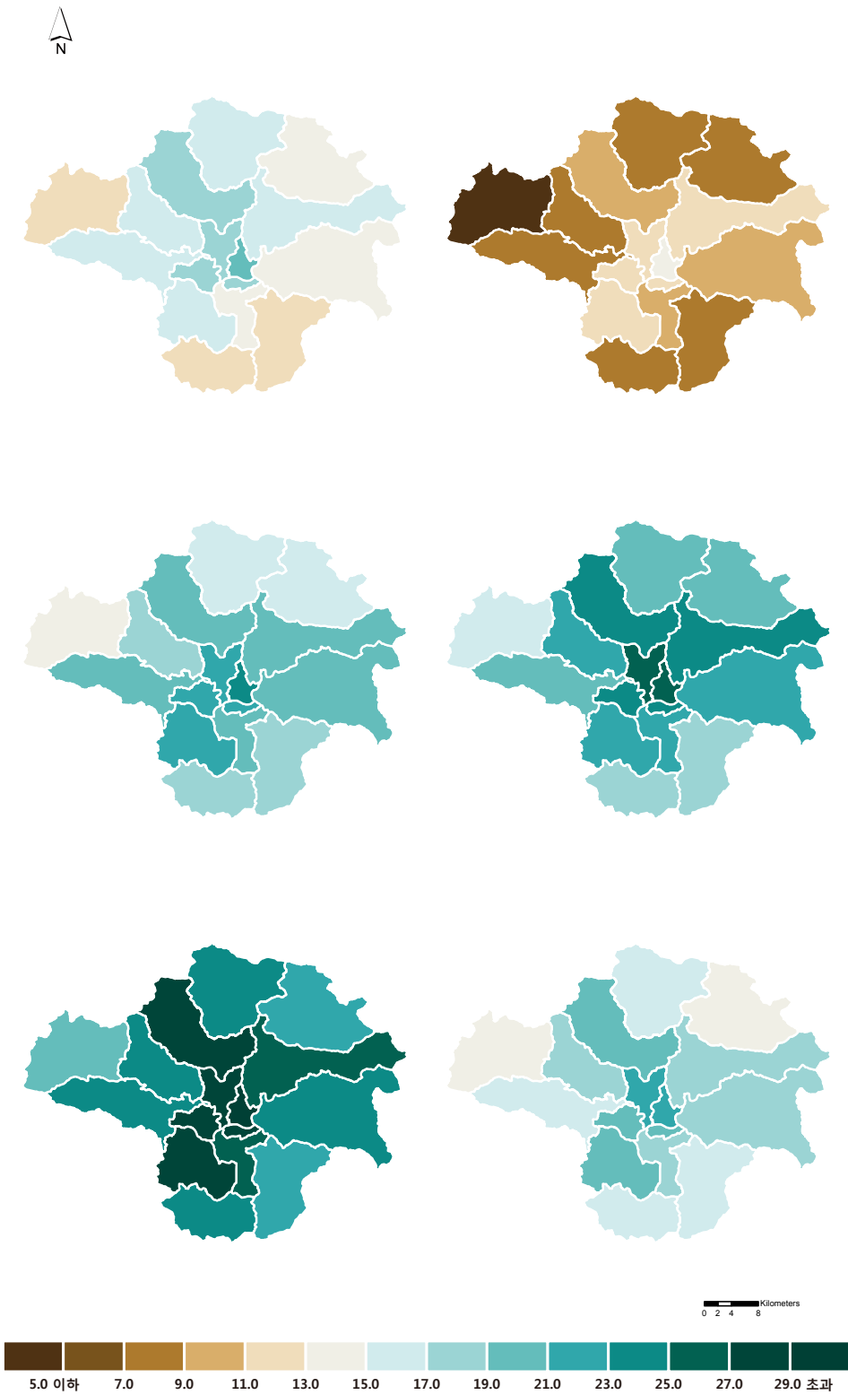
그림 3-7. 영천시의 읍면동별 강수량 증가율(%) (2001~2010년 대비) 분포도 (RCP4.5(좌)/8.5(우), 2011~2040년(상), 2041~2070년(중), 2071~2100년(하))
