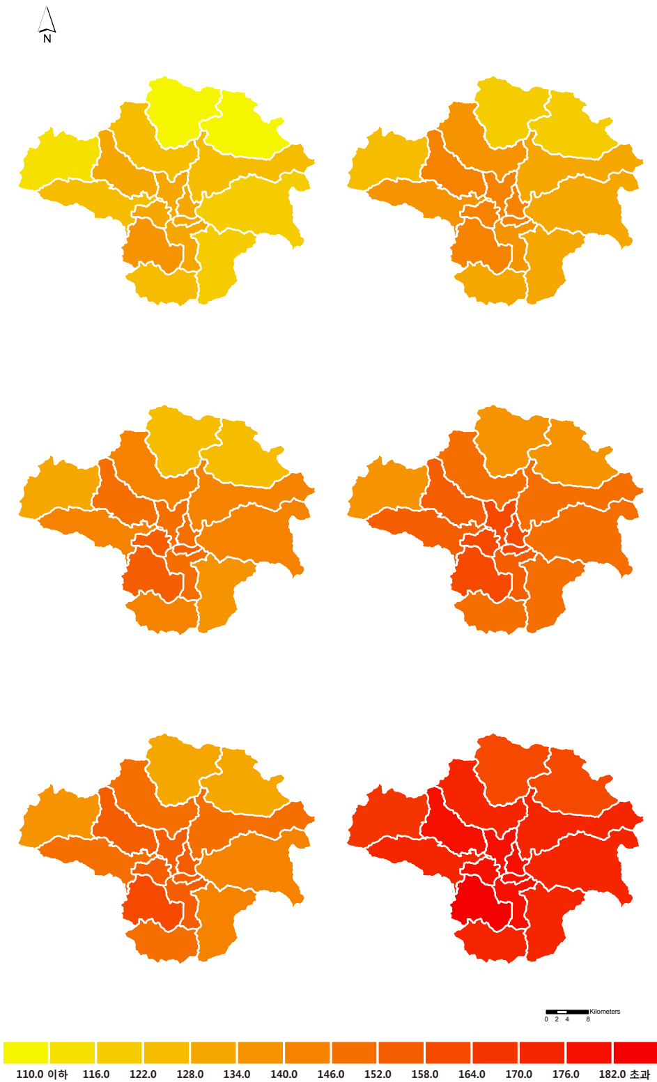
그림 3-13. 영천시 읍면동별 여름일수(일) 분포도 (RCP4.5(좌)/8.5(우), 2011~2040년(상), 2041~2070년(중), 2071~2100년(하))
