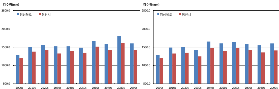
그림 3-4. 경상북도과 영천시와 연강수량(mm) 시계열 (RCP4.5(좌), RCP8.5(우))
