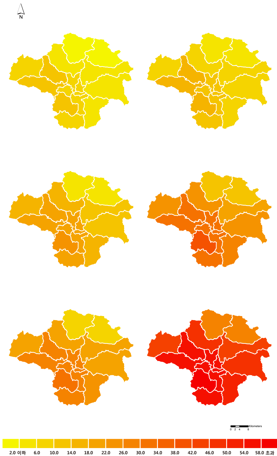
그림 3-9. 영천시읍면동별 열대야일수(일) 분포도 (RCP4.5(좌)/8.5(우), 2011~2040년(상), 2041~2070년(중), 2071~2100년(하))
