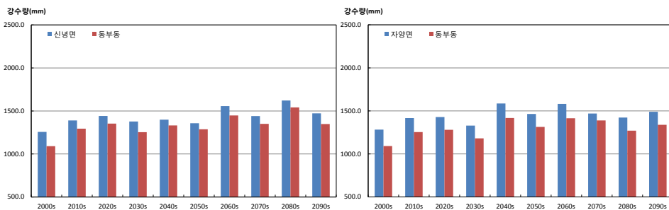
그림 3-5. 연강수량(mm) 증가율이 가장 큰 지역 (동부동)과 작은 지역(신녕면, 자양면)의 시계열 (RCP4.5(좌), RCP8.5(우))
