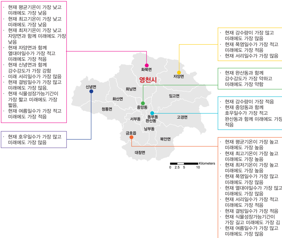
그림 5-1. 경상북도 영천시의 읍면동별 기후변화 전망 요약
