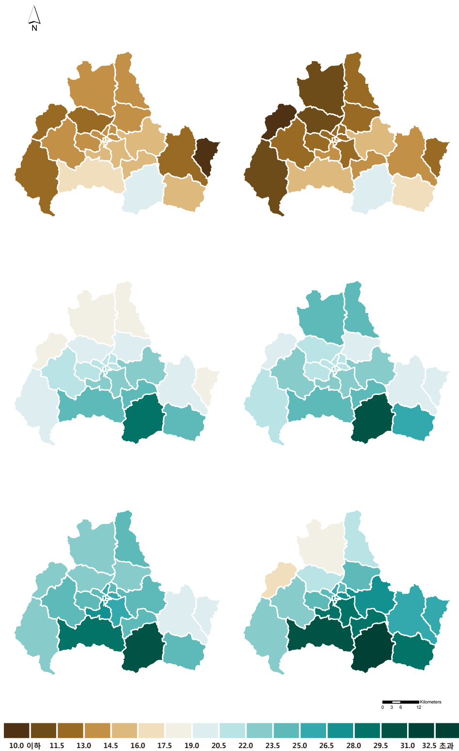
그림 3-7. 경주시의 읍면동별 강수량 증가율(%) (2001~2010년 대비) 분포도 (RCP4.5(좌)/8.5(우), 2011~2040년(상), 2041~2070년(중), 2071~2100년(하))
