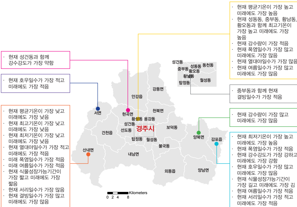
그림 5-1. 경상북도 경주시의 읍면동별 기후변화 전망 요약
