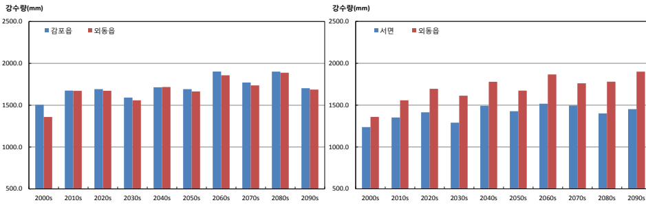
그림 3-5. 연강수량(mm) 증가율이 가장 큰 지역(외동읍)과 작은 지역(감포읍, 서면)의 시계열 (RCP4.5(좌), RCP8.5(우))
