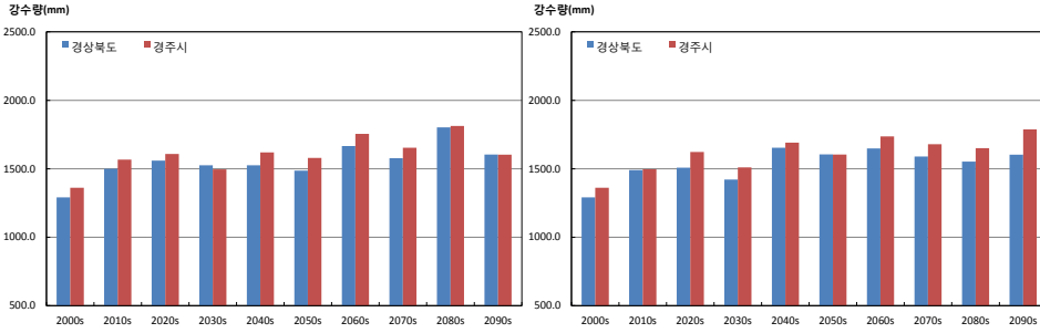
그림 3-4. 경상북도와 경주시의 연강수량(mm) 시계열 (RCP4.5(좌), RCP8.5(우))
