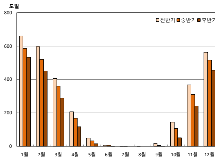
그림 4-6. 김천시의 월별 난방도일(도일) 전망 (RCP4.5(좌), RCP8.5(우))
