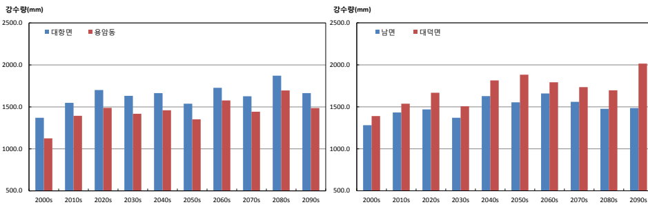
그림 3-5. 연강수량(mm) 증가율이 가장 큰 지역 (Yungam-dong, Daedakmyeon)과 작은 지역(Daehangmyeon, Nammyeon)의 시계열 (RCP4.5(좌), RCP8.5(우))
