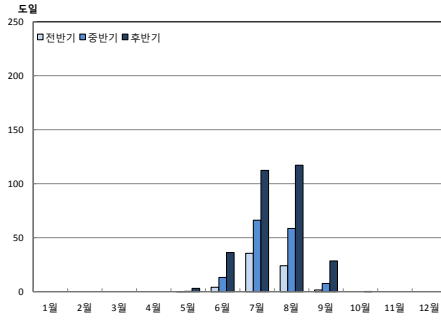
그림 4-5. 김천시의 월별 냉방도일(도일)전망 (RCP4.5(좌), RCP8.5(우))
