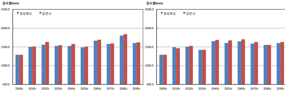
그림 3-4. 경상북도와 김천시의 연강수량(mm) 시계열 (RCP4.5(좌), RCP8.5(우))
