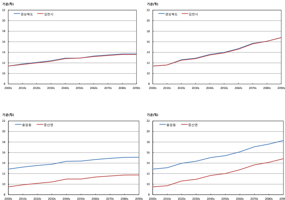
그림 3-1. 경상북도와 김천시의 평균기온(℃) 시계열(RCP4.5(좌), RCP8.5(우))
