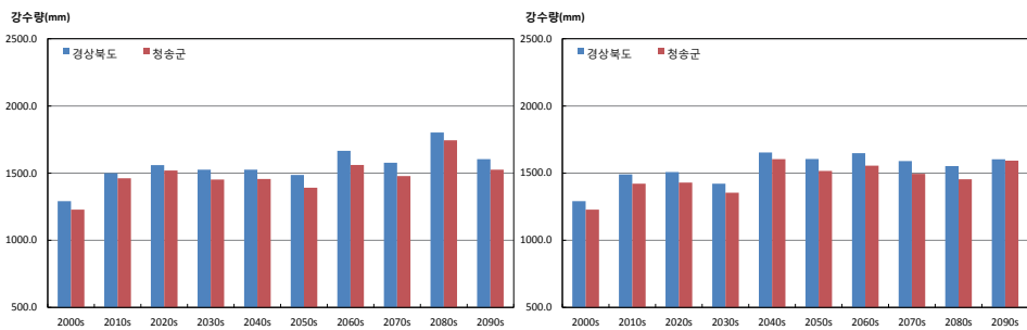
그림 3-4. 경상북도와 청송군의 연강수량(mm) 시계열 (RCP4.5(좌), RCP8.5(우))
