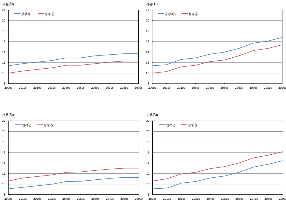
그림 3-1. 경상북도과 청송군의 평균기온(℃) 시계열(RCP4.5(좌), RCP8.5(우))
