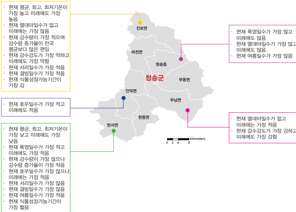
그림 5-1. 경상북도 청송군의 읍면별 기후변화 전망 요약
