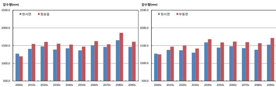
그림 3-5. 연강수량(mm) 증가율이 가장 큰 지역 (청송읍, 부동면)과 작은 지역(현서면)의 시계열 (RCP4.5(좌), RCP8.5(우))
