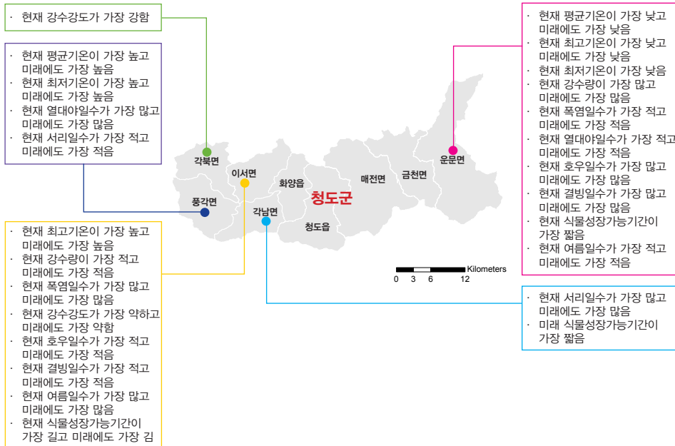
그림 5-1. 경상북도 청도군의 읍면별 기후변화 전망 요약
