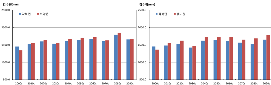
그림 3-5. 연강수량(mm) 증가율이 가장 큰 지역 (화양읍, 청도읍)과 작은 지역(각북면)의 시계열 (RCP4.5(좌), RCP8.5(우))
