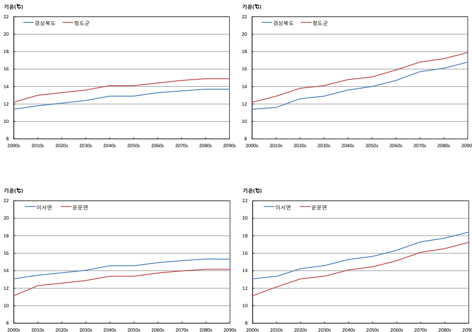
그림 3-1. 경상북도와 청도군의 평균기온(℃) 시계열(RCP4.5(좌), RCP8.5(우))
