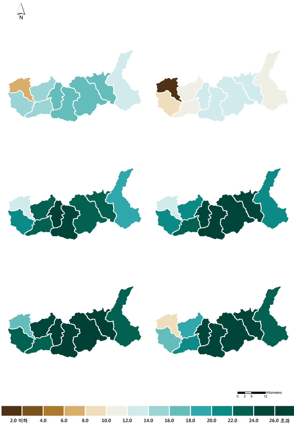
그림 3-7. 청도군의 읍면별 강수량 증가율(%) (2001~2010년 대비) 분포도 (RCP4.5(좌)/8.5(우), 2011~2040년(상), 2041~2070년(중), 2071~2100년(하))
