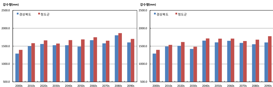
그림 3-4. 경상북도와 청도군의 연강수량(mm) 시계열 (RCP4.5(좌), RCP8.5(우))
