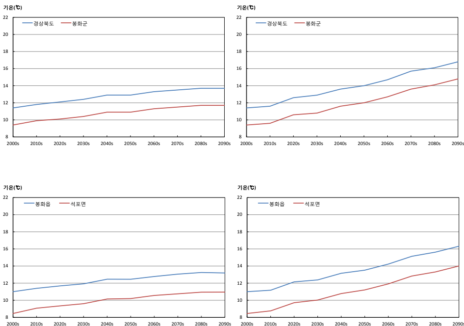
그림 3-1. 경상북도와 봉화군의 평균기온(℃) 시계열(RCP4.5(좌), RCP8.5(우))
