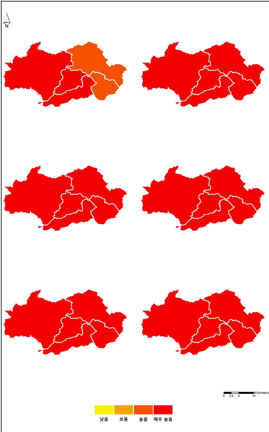
그림 4-4. 광주광역시 구별 불래지수 분포도 (RCP4.5(좌)/8.5(우), 2011~2040년(상), 2041~2070년(중), 2071~2100년(하))
