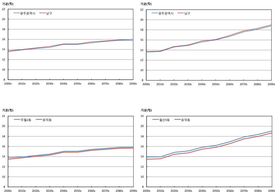
그림 3-1. 광주광역시와 남구의 평균기온(℃) 시계열(RCP4.5(좌), RCP8.5(우))
