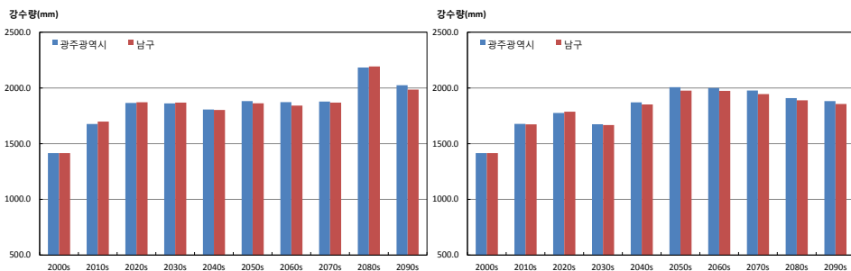
그림 3-4. 광주광역시와 남구의 연강수량(mm) 시계열 (RCP4.5(좌), RCP8.5(우))
