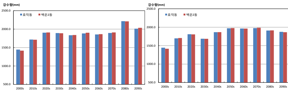
그림 3-5. 연강수량(mm) 증가율이 가장 큰 지역 (백운2동)과 작은 지역(효덕동)의 시계열 (RCP4.5(좌), RCP8.5(우))
