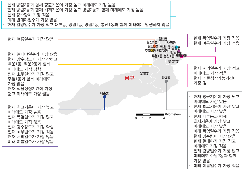
그림 5-1. 광주광역시 남구의 동별 기후변화 전망 요약
