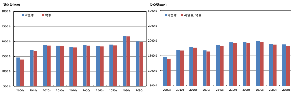
그림 3-5. 연강수량(mm) 증가율이 가장 큰 지역 (학동, 서남동)과 작은 지역(학운동)의 시계열(RCP4.5(좌), RCP8.5(우))
