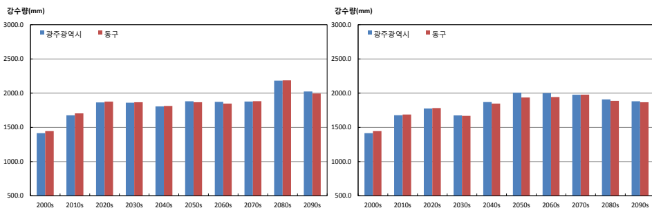
그림 3-4. 광주광역시와 동구의 연강수량(mm) 시계열 (RCP4.5(좌), RCP8.5(우))
