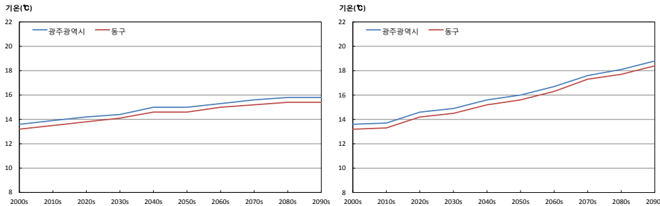
그림 3-1. 광주광역시와 동구의 평균기온(℃) 시계열(RCP4.5(좌), RCP8.5(우))
