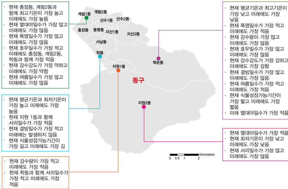
그림 5-1. 광주광역시 동구의 동별 기후변화 전망 요약(RCP8.5 2071~2100년)
