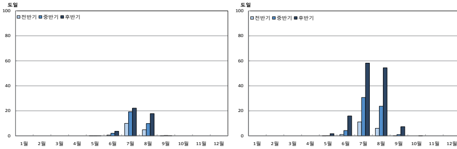
그림 4-5. 양양군의 월별 냉방도일(도일)전망 (RCP4.5(좌), RCP8.5(우))
