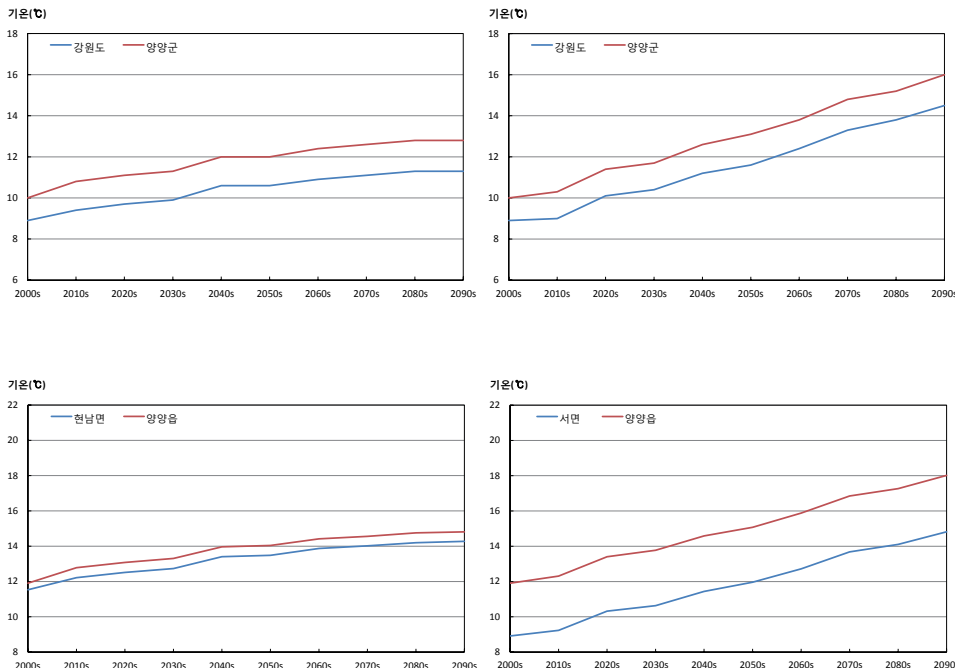
그림 3-1. 강원도와 양양군의 평균기온(℃) 시계열(RCP4.5(좌), RCP8.5(우))
