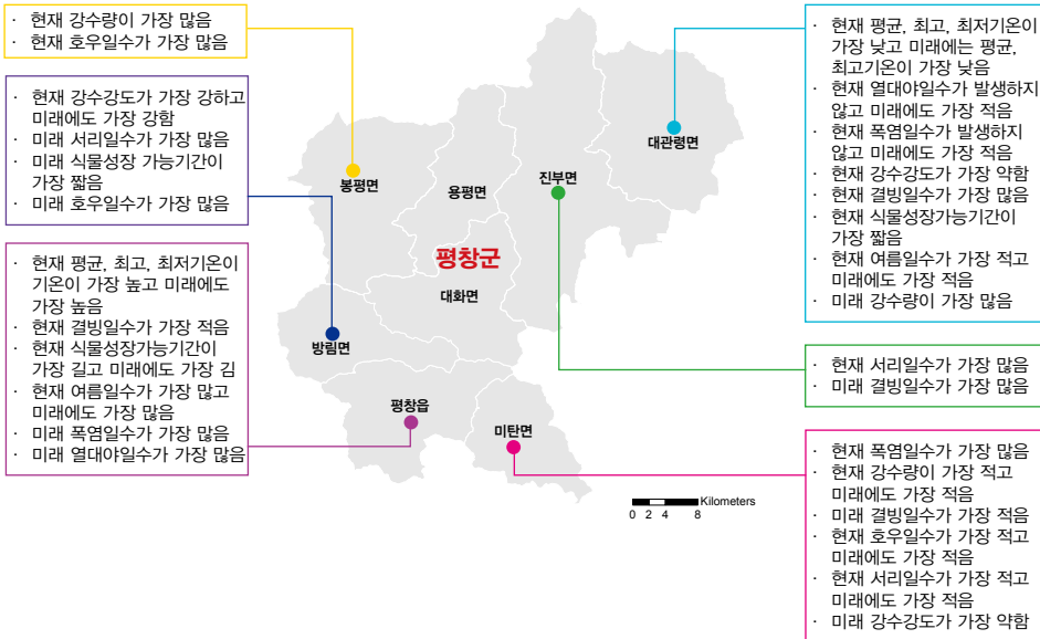
그림 5-1. 강원도 평창군의 읍면별 기후변화 전망 요약(RCP8.5 2071~2100년)
