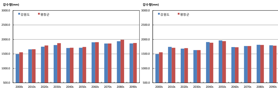
그림 3-4. 강원도와 평창군의 연강수량(mm) 시계열 (RCP4.5(좌), RCP8.5(우))
