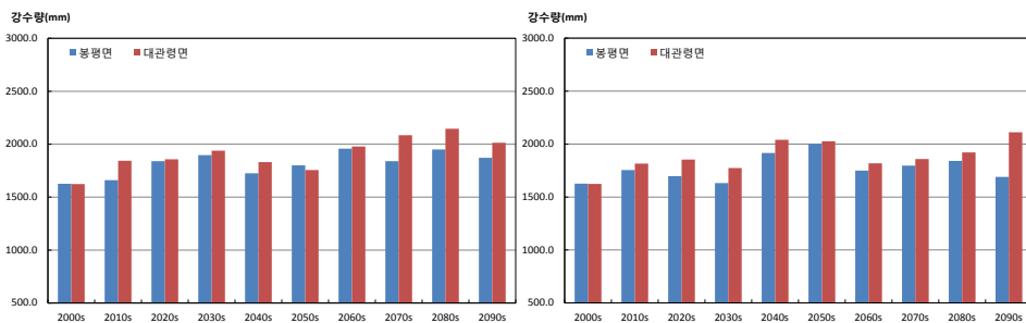
그림 3-5. 연강수량(mm) 증가율이 가장 큰 지역 (대관령면)과 작은 지역(봉평면)의 시계열 (RCP4.5(좌), RCP8.5(우))
