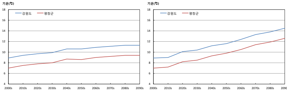
그림 3-1. 강원도와 평창군의 평균기온(℃) 시계열(RCP4.5(좌), RCP8.5(우))
