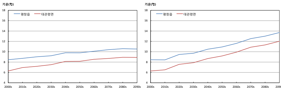
그림 3-2. 평균기온(℃) 증가율이 가장 큰 지역(대관령면)과 작은 지역(평창읍)의 시계열(RCP4.5(좌), RCP8.5(우))
