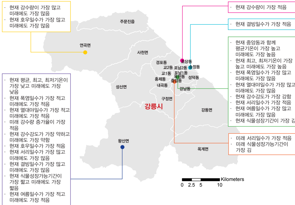
그림 5-1. 강원도 강릉시의 읍면동별 기후변화 전망 요약
