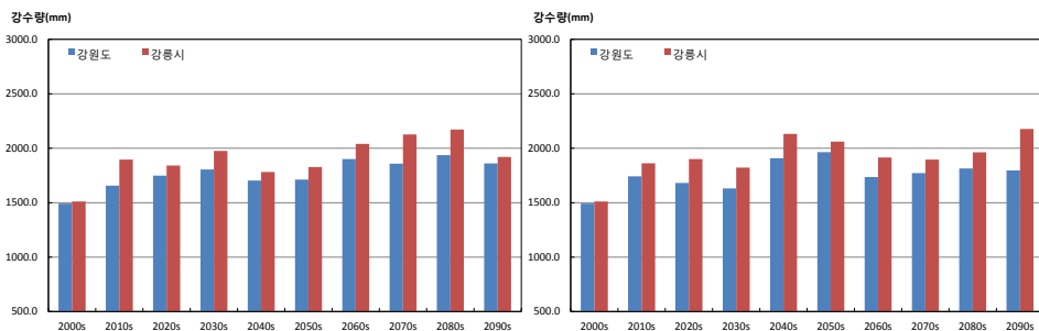
그림 3-4. 강원도와 강릉시의 연강수량(mm) 시계열 (RCP4.5(좌), RCP8.5(우))
