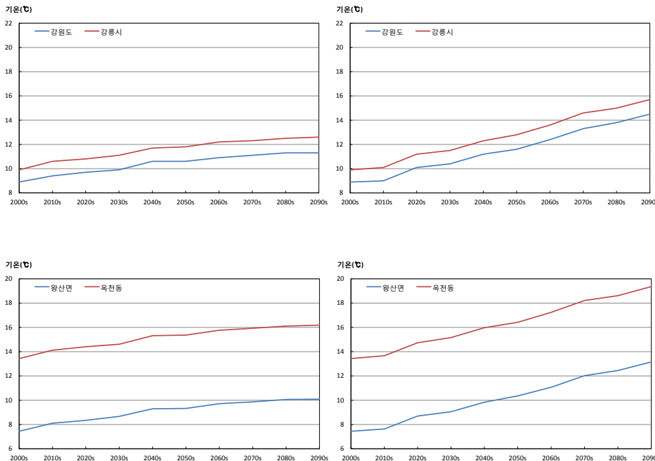
그림 3-1. 강원도와 강릉시의 평균기온(℃) 시계열(RCP4.5(좌), RCP8.5(우))
