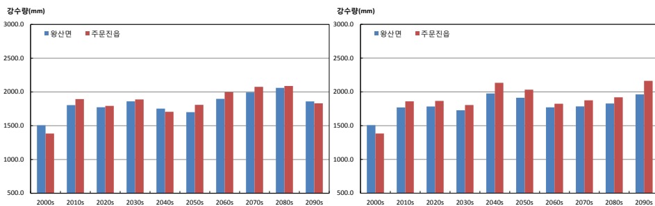
그림 3-5. 연강수량(mm) 증가율이 가장 큰 지역 (주문진읍)과 작은 지역(왕산면)의 시계열 (RCP4.5(좌), RCP8.5(우))
