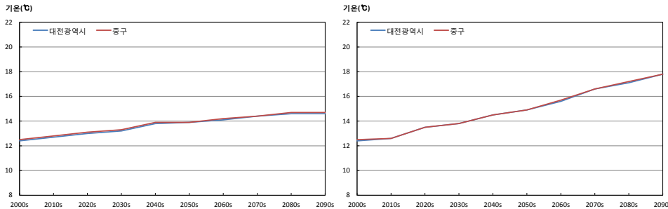
그림 3-1. 대전광역시와 중구의 평균기온(℃) 시계열(RCP4.5(좌), RCP8.5(우))
