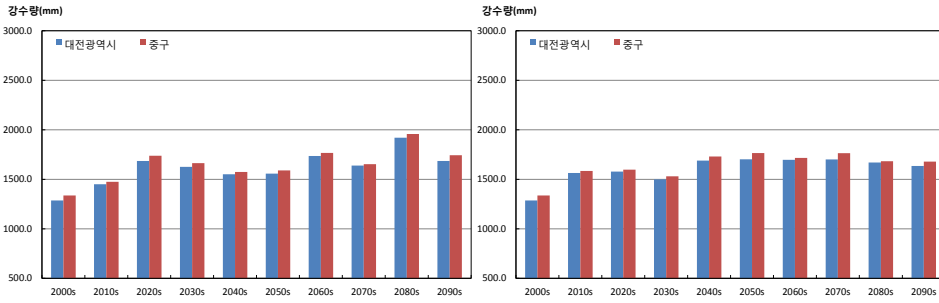
그림 3-4. 대전광역시와 중구의 연강수량(mm) 시계열 (RCP4.5(좌), RCP8.5(우))
