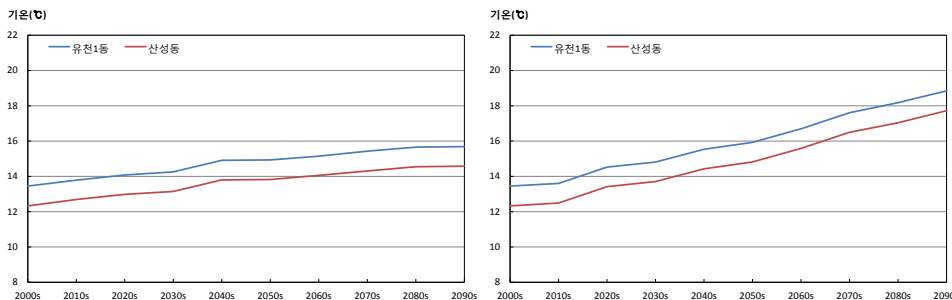
그림 3-2. 평균기온(℃) 증가율이 가장 큰 지역 (산성동)과 작은 지역(유천1동)의 시계열(RCP4.5(좌), RCP8.5(우))
