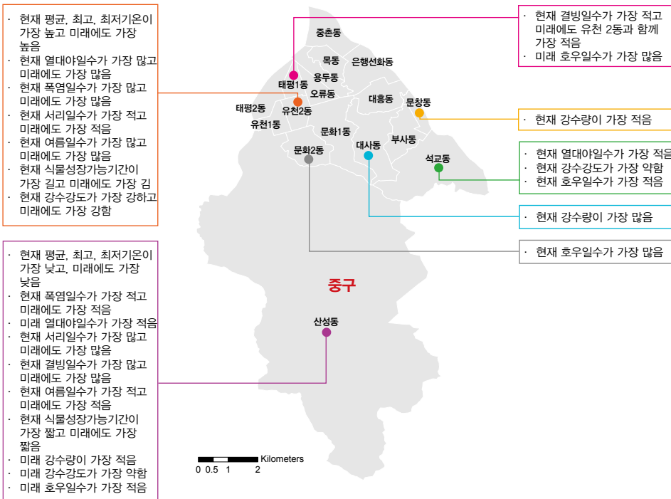
그림 5-1. 대전광역시 중구의 동별 기후변화 전망 요약(RCP8.5 2071~2100년)
