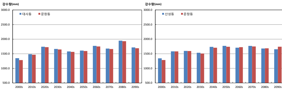
그림 3-5. 연강수량(mm) 증가율이 가장 큰 지역 (문창동)과 작은 지역(대사동, 산성동)의 시계열 (RCP4.5(좌), RCP8.5(우))
