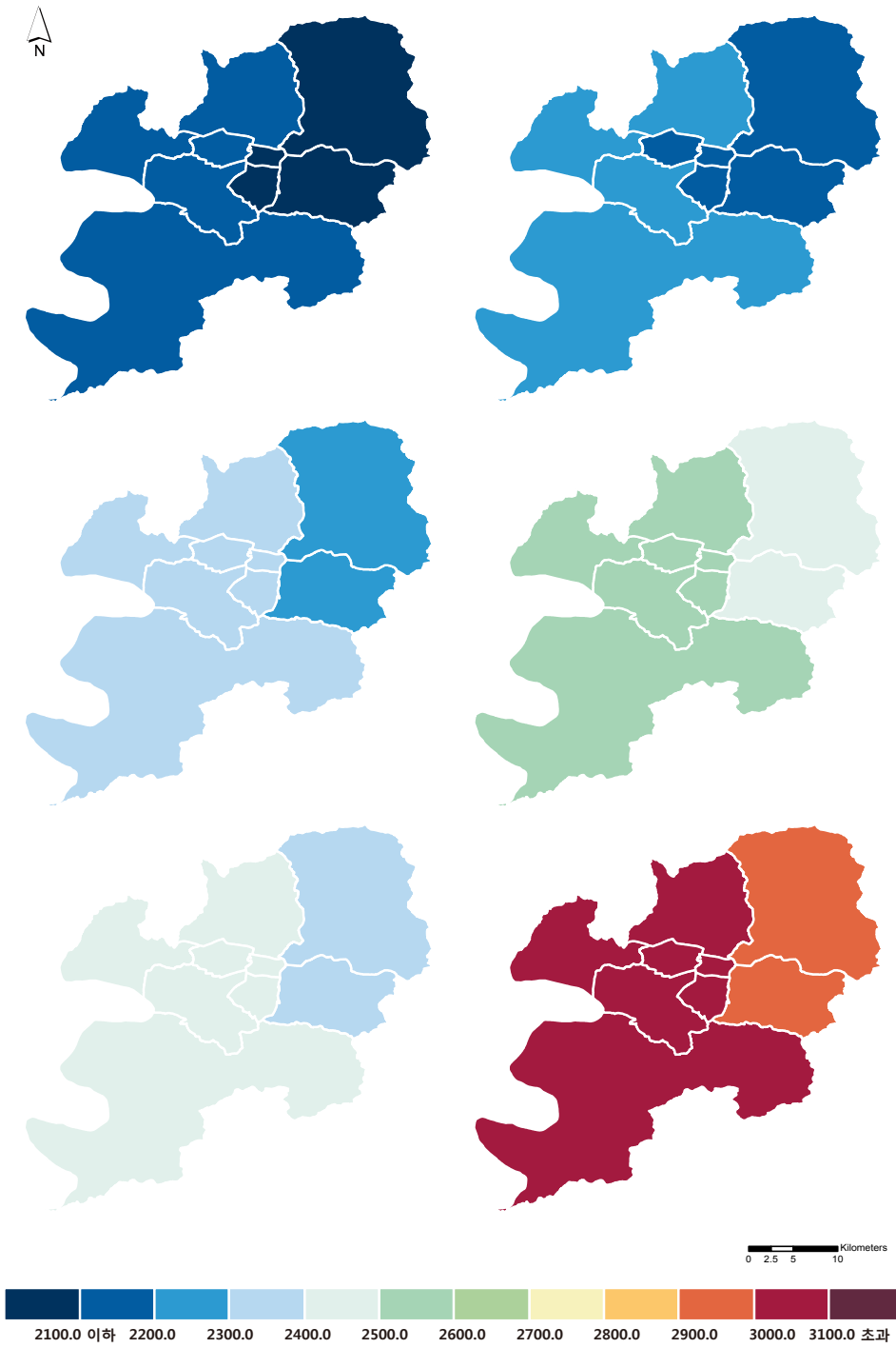
그림 4-2. 대구광역시 구군별 유효적산온도(10°C)(°C) 분포도 (RCP4.5(좌)/8.5(우), 2011~2040년(상), 2041~2070년(중), 2071~2100년(하))
