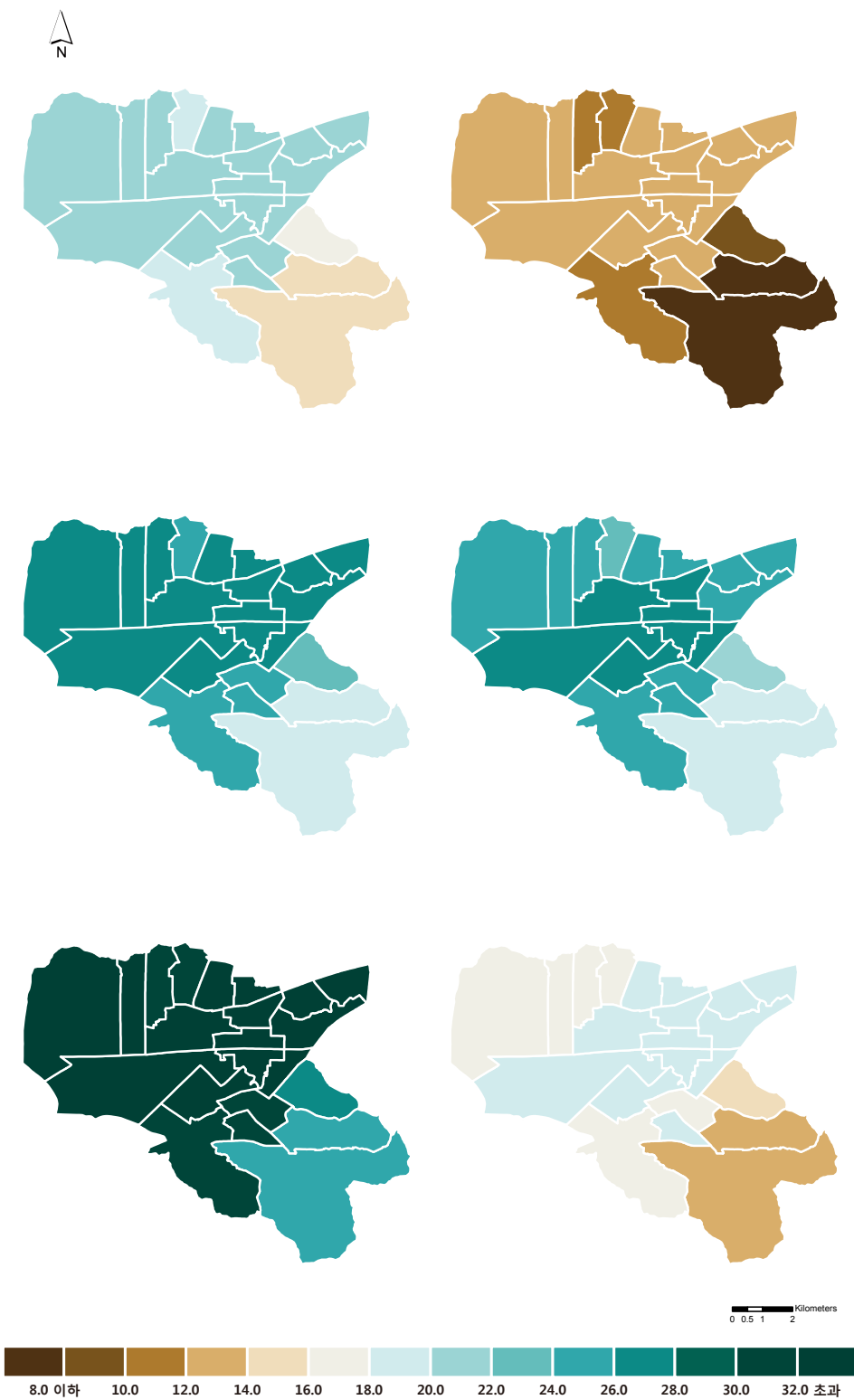
그림 3-7. 달서구의 동별 강수량 증가율(%) (2001~2010년 대비) 분포도 (RCP4.5(좌)/8.5(우), 2011~2040년(상), 2041~2070년(중), 2071~2100년(하))
