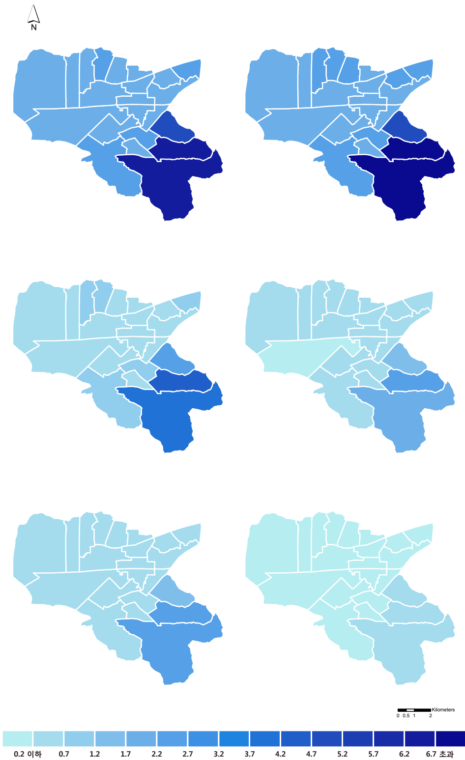
그림 3-11. 달서구의 동별 결빙일수(일) 분포도 (RCP4.5(좌)/8.5(우), 2011~2040년(상), 2041~2070년(중), 2071~2100년(하))
