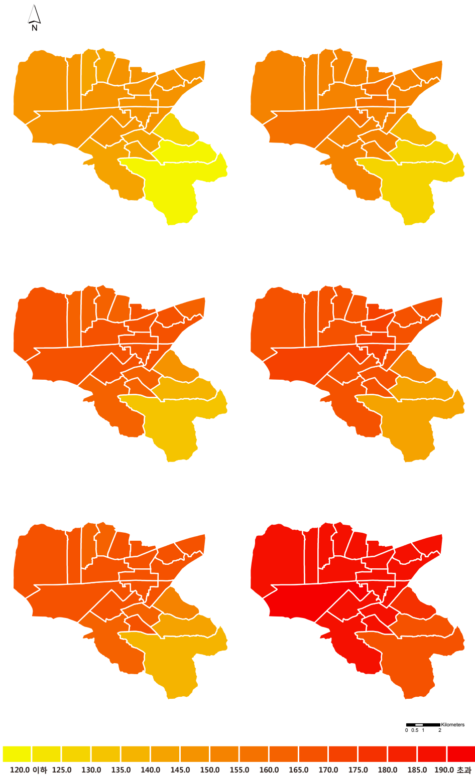
그림 3-13. 달서구의 동별 여름일수(일) 분포도 (RCP4.5(좌)/8.5(우), 2011~2040년(상), 2041~2070년(중), 2071~2100년(하))
