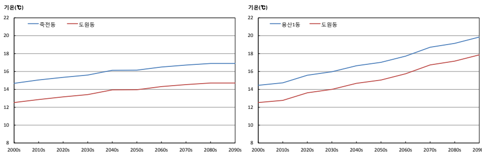
그림 3-2. 평균기온(℃) 증가율이 가장 큰 지역 (도원동)과 작은 지역(죽전동, 용산1동)의 시계열(RCP4.5(좌), RCP8.5(우))
