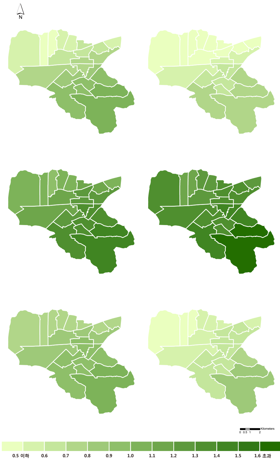
그림 3-15. 달서구의 동별 호우일수(일) 분포도 (RCP4.5(좌)/8.5(우), 2011~2040년(상), 2041~2070년(중), 2071~2100년(하))
