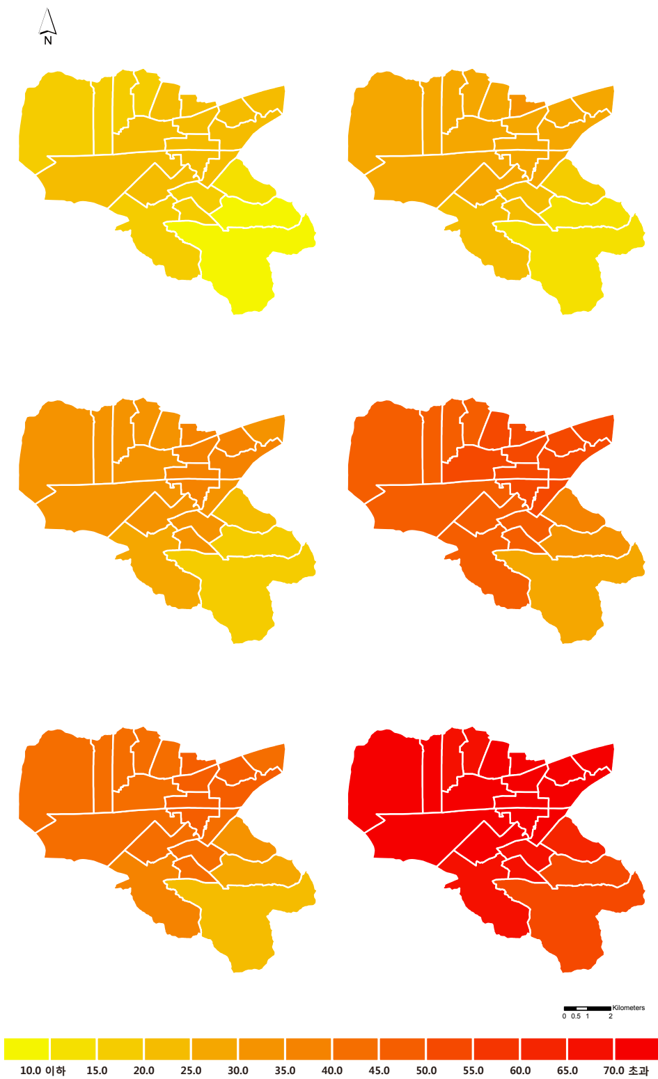
그림 3-9. 달서구의 동별 열대야일수(일) 분포도 (RCP4.5(좌)/8.5(우), 2011~2040년(상), 2041~2070년(중), 2071~2100년(하))
