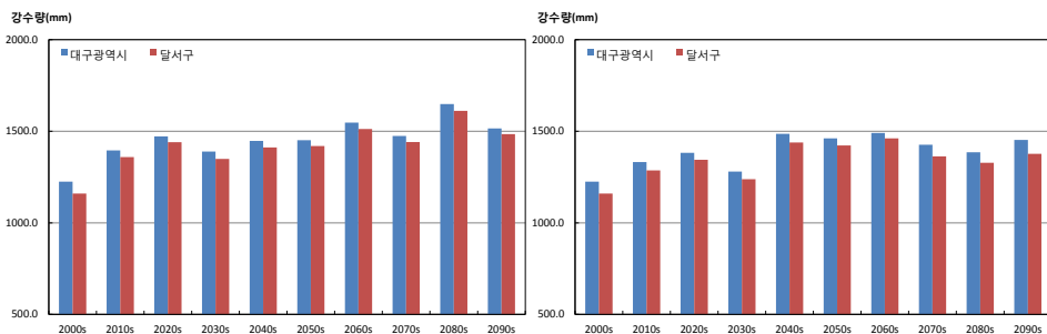
그림 3-4. 대구광역시와 달서구의 연강수량(mm) 시계열 (RCP4.5(좌), RCP8.5(우))
