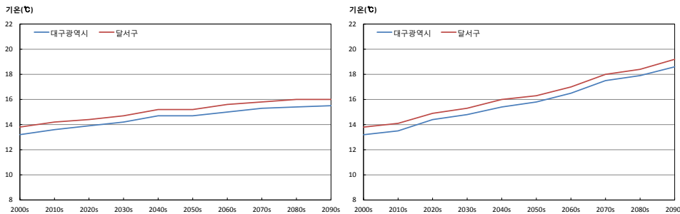
그림 3-1. 대구광역시와 달서구의 평균기온(℃) 시계열(RCP4.5(좌), RCP8.5(우))
