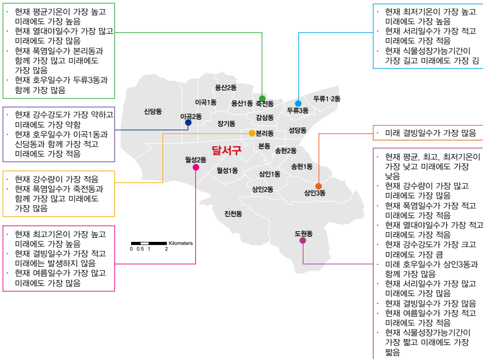
그림 5-1. 대구광역시 달서구의 동별 기후변화 전망 요약(RCP8.5 2071~2100년)
