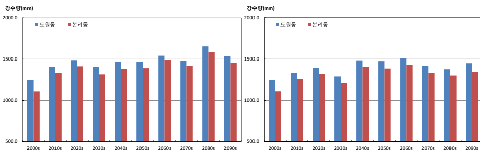
그림 3-5. 연강수량(mm) 증가율이 가장 큰 지역 (본리동)과 작은 지역(도원동)의 시계열(RCP4.5(좌), RCP8.5(우))
