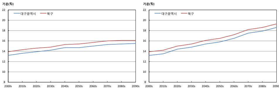
그림 3-1. 대구광역시와 북구의 평균기온(℃) 시계열(RCP4.5(좌), RCP8.5(우))
