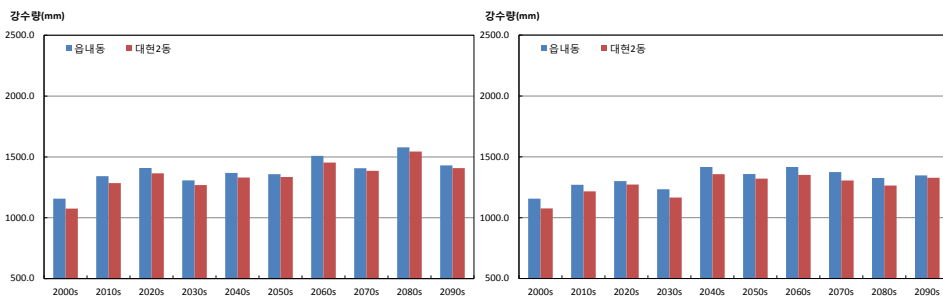
그림 3-5. 연강수량(mm) 증가율이 가장 큰 지역 (대현2동)과 작은 지역(읍내동)의 시계열(RCP4.5(좌), RCP8.5(우))
