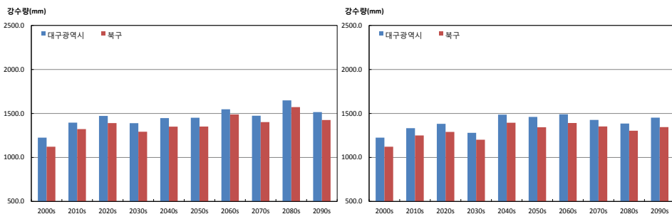
그림 3-4. 대구광역시의 북구의 연강수량(mm) 시계열 (RCP4.5(좌), RCP8.5(우))
