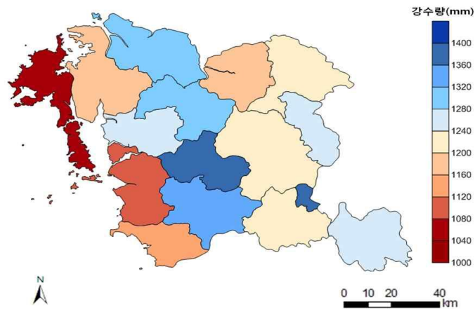
그림 2-2. 충청남도의 행정구역별 연강수량 상세분포도(2001~2010년)
