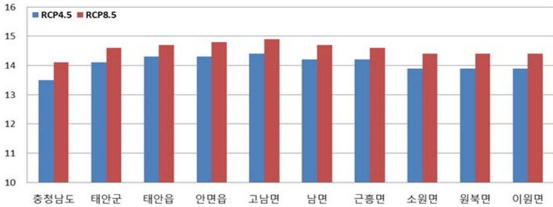
그림 3-3. 2040s의 읍면동별 평균기온 RCP 4.5(청), RCP 8.5(적)
