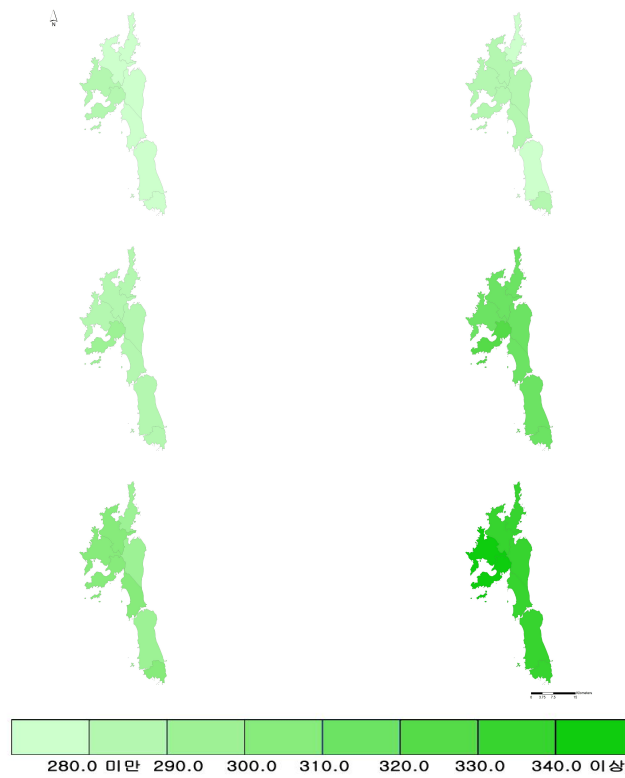
그림 3-14. RCP 4.5(좌)/8.5(우) 식물성장가능기간 분포도 (2011~2040년(상), 2041~2070년(중), 2071~2100년(하))
