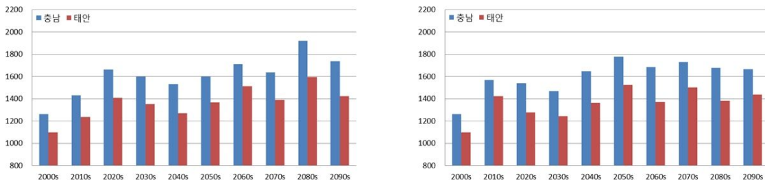
그림 3-4. 충청남도과 태안군의 연강수량 시계열 RCP 4.5(좌), RCP 8.5(우)
