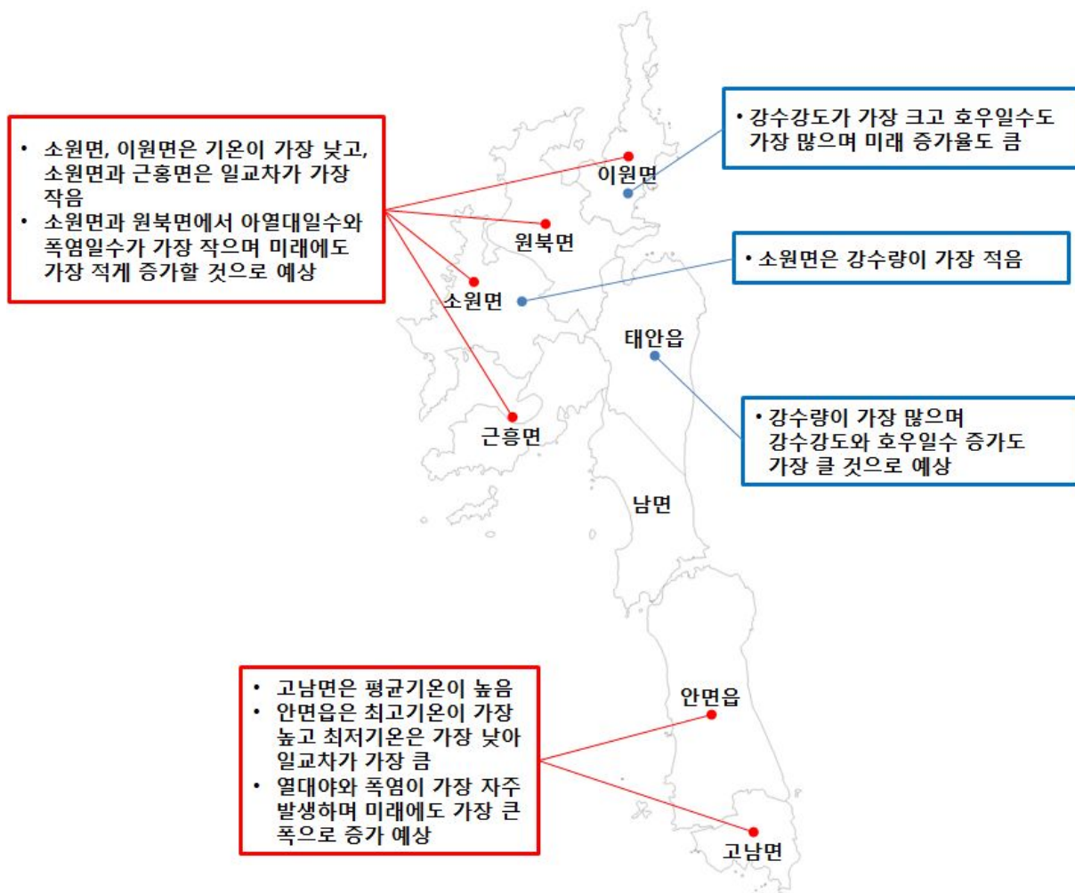
그림 4-1. 충청남도 태안군 동별 기후변화 전망 요약
