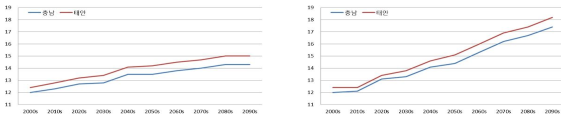
그림 3-1. 충청남도과 태안군의 평균기온 시계열 RCP 4.5(좌), RCP 8.5(우)
